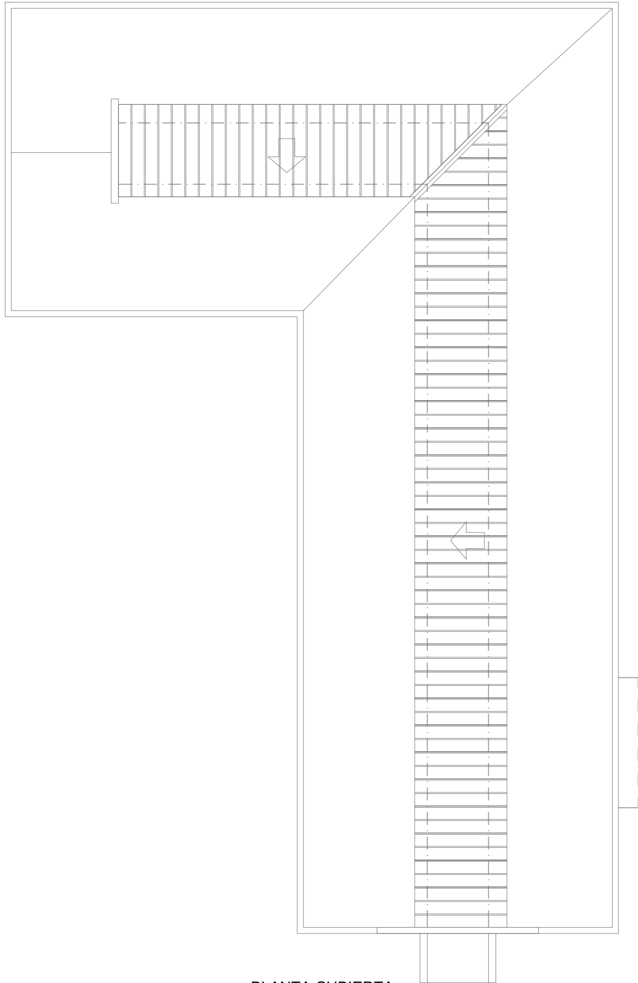
PLANTA CUBIERTA
