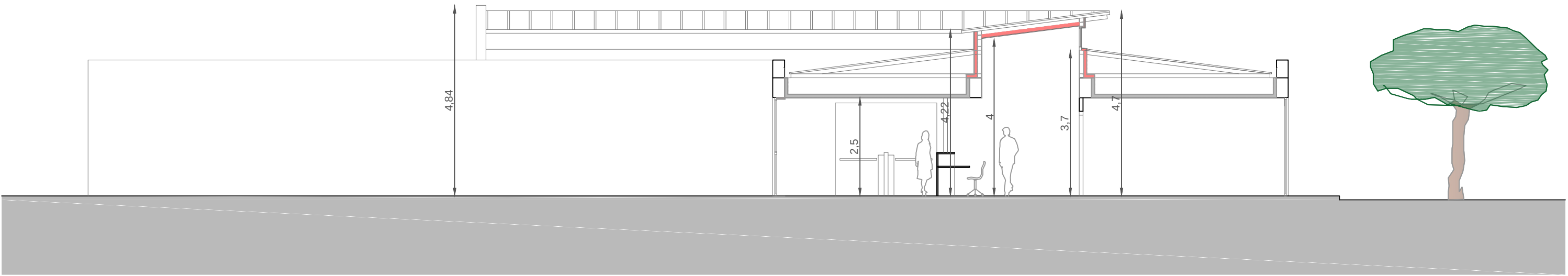
SECCIÓN A-A' _ ACCESO PISCINAS _ ESTADO REFORMADO
