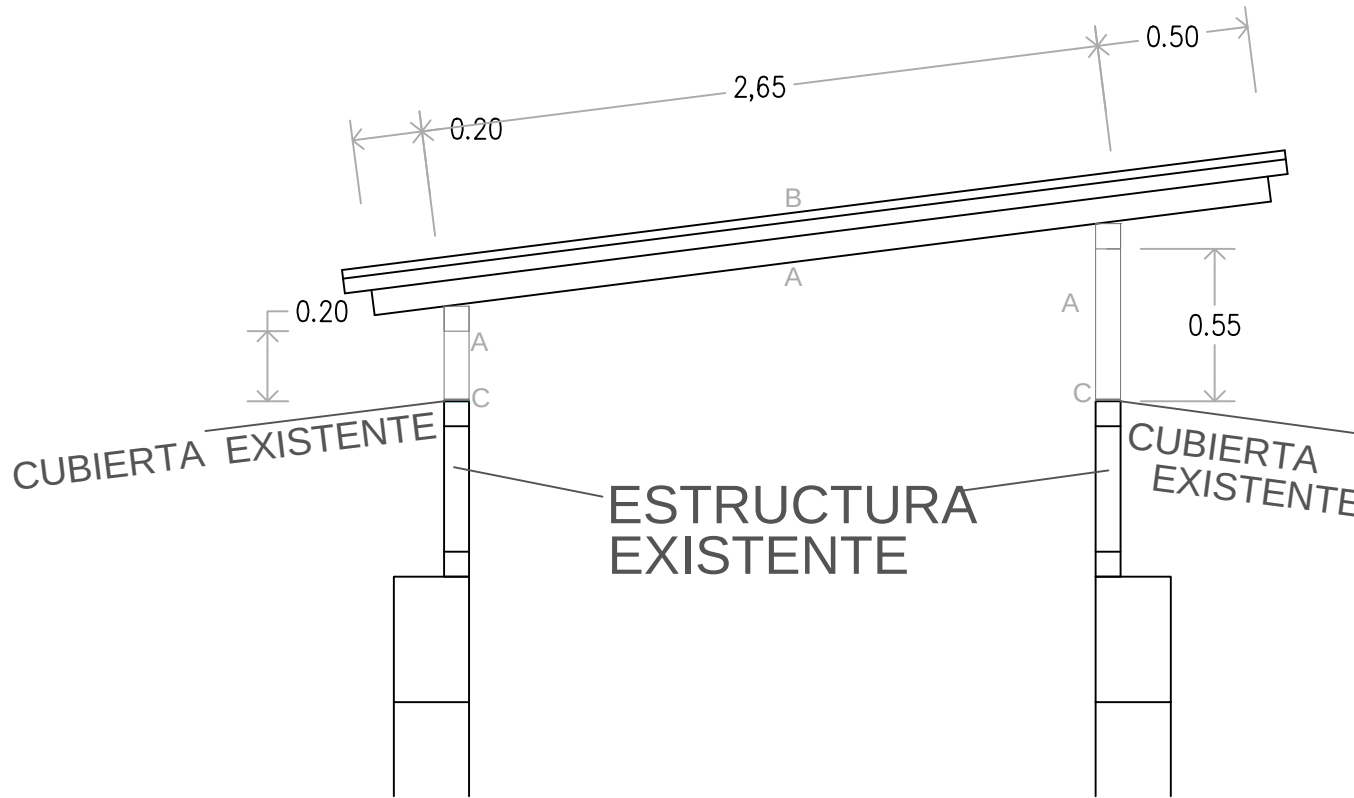
DETALLE ESTRUCTURA METÁLICA CLARABOYA
