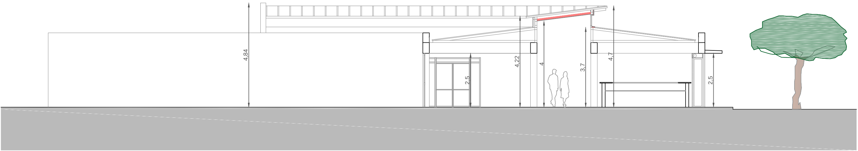
SECCIÓN B-B' _ BAR _ ESTADO REFORMADO
