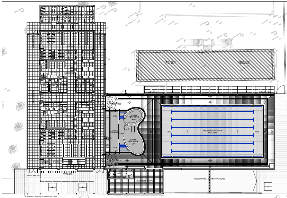
Plano Piscinas y Vestuarios (Fase 1 proyecto)
