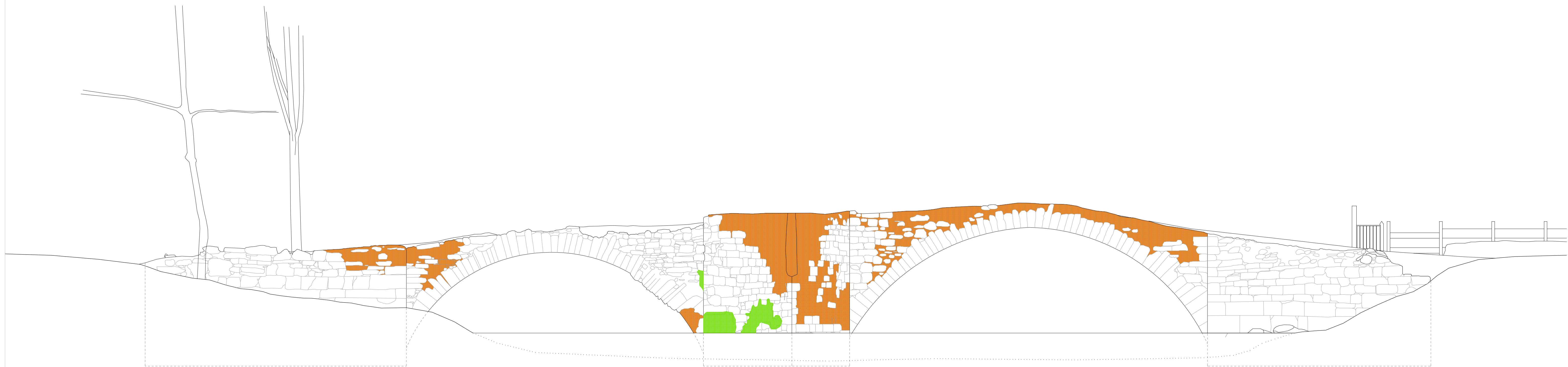
Alzado Aguas Arriba
