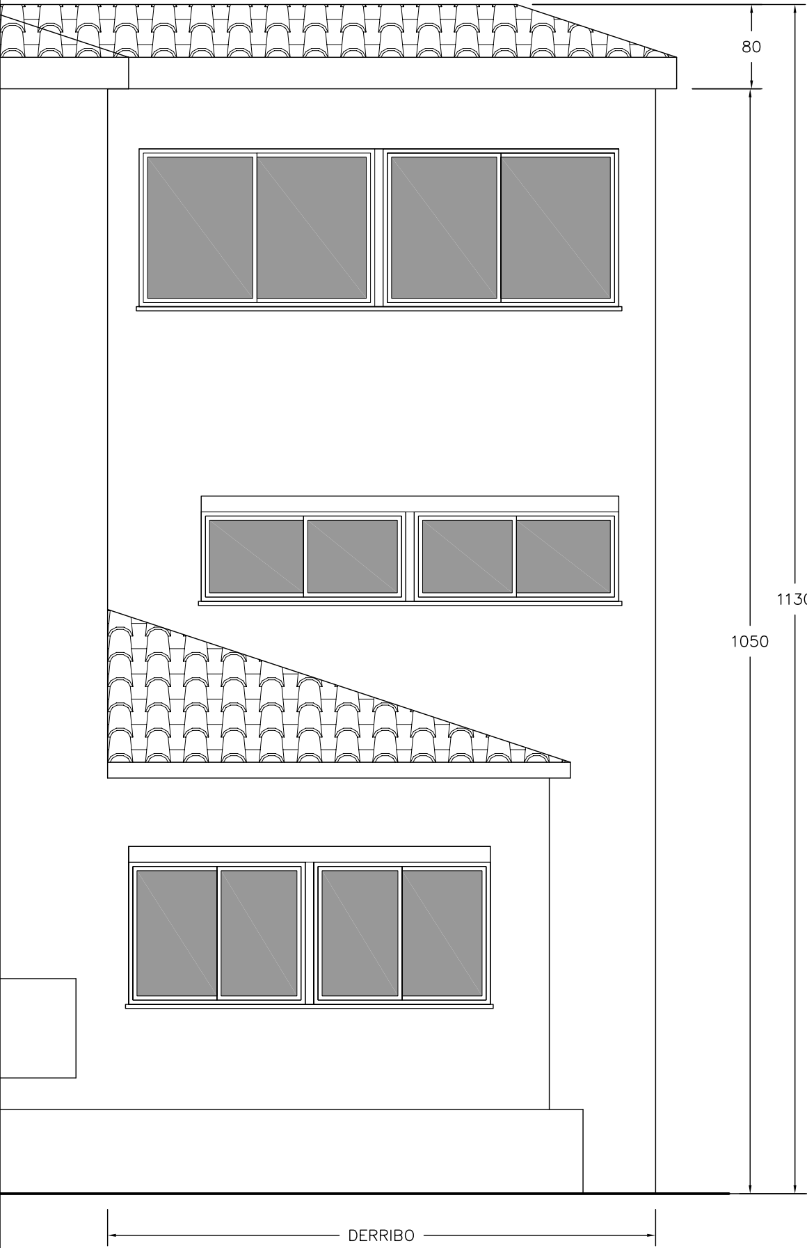
ALZADO ESTE
