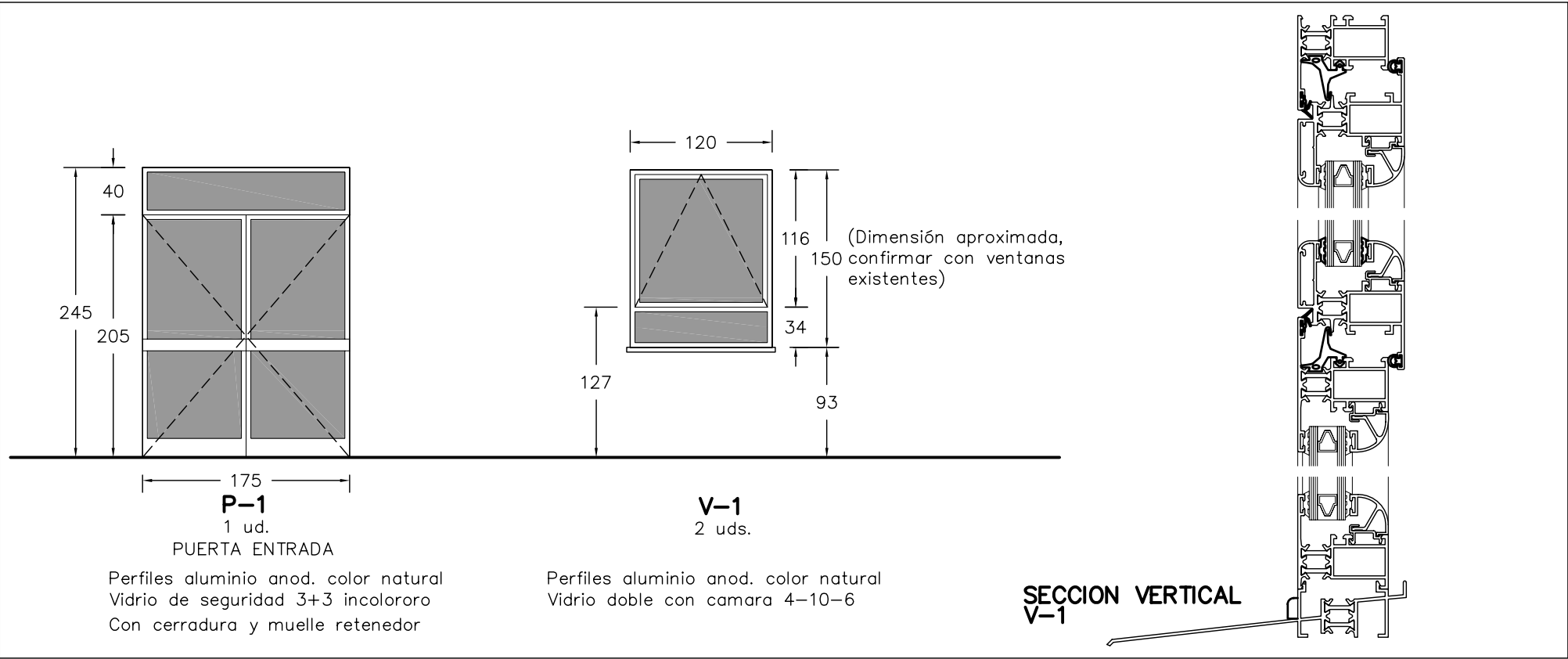
ALZADO ESTE
