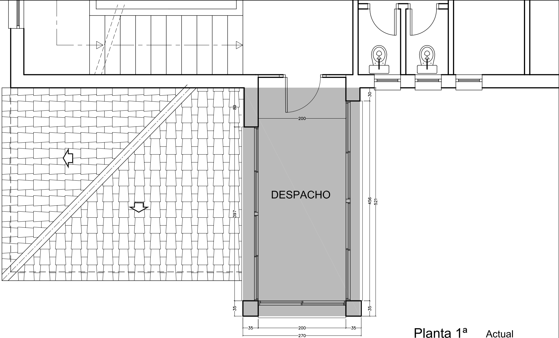
Planta 1ª Actual
