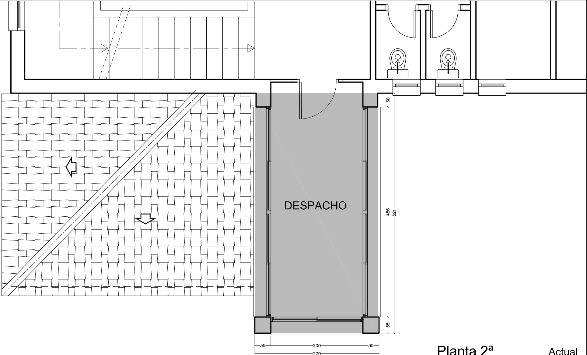
Planta 2ª Actual
