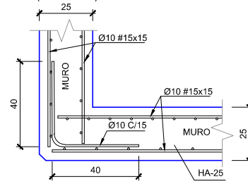
SECCIÓN PARCIAL HORIZONTAL VISTA EN PLANTA (ENCUENTRO DE MUROS)
