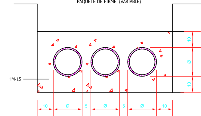
SECCIÓN TIPO CANALIZACIÓN
