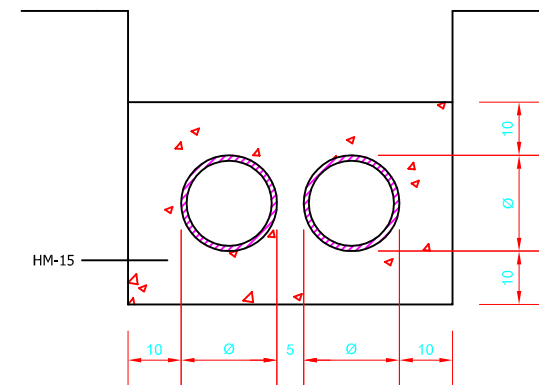
SECCIÓN TIPO CANALIZACIÓN
