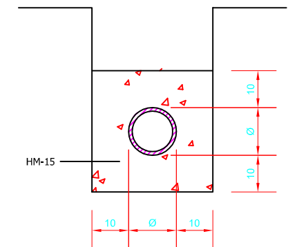
SECCIÓN TIPO CANALIZACIÓN
