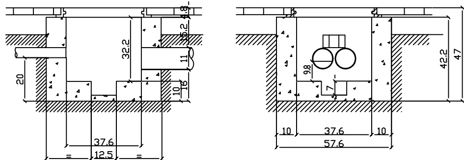
Arqueta tipo 40X40
