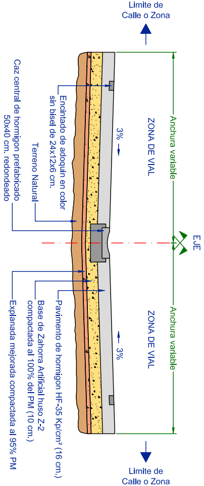
SECCION E: 1/50
