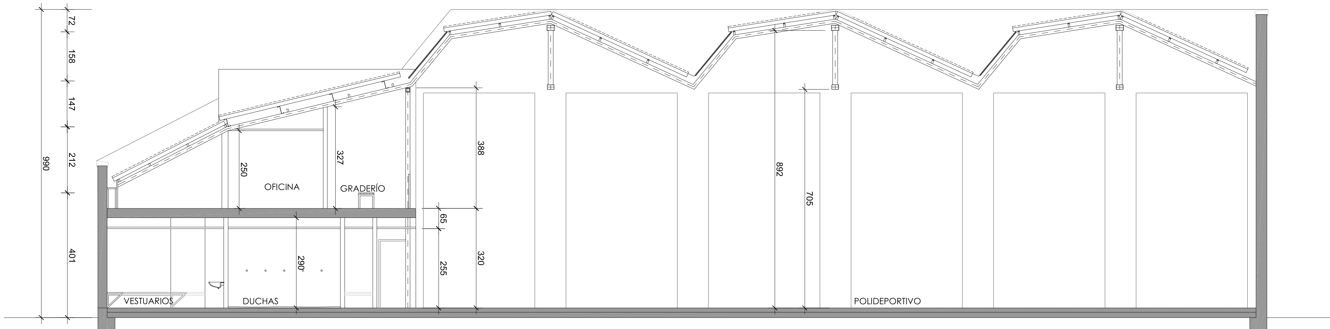
SECCION TRANSVERSAL
