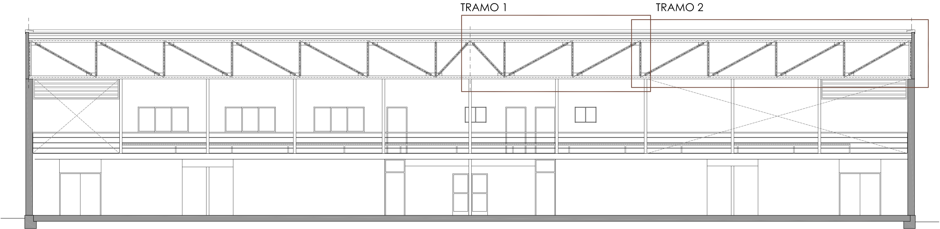
SECCIÓN LONGITUDINAL
