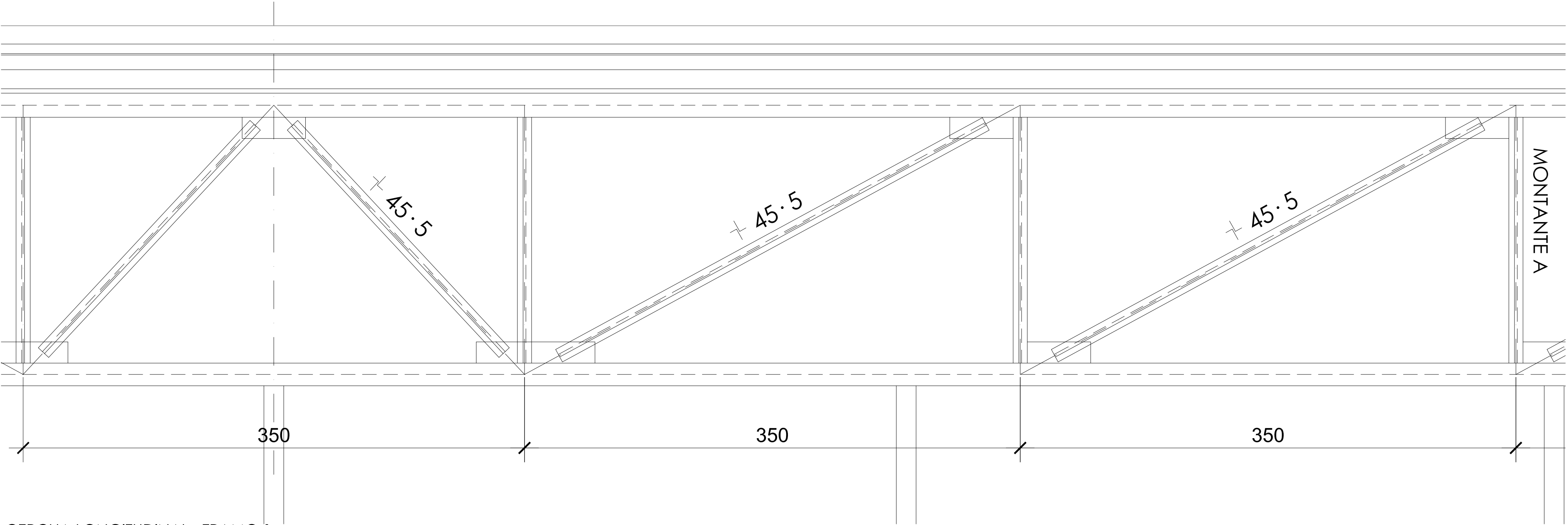
CERCHA LONGITUDINAL - TRAMO 1
