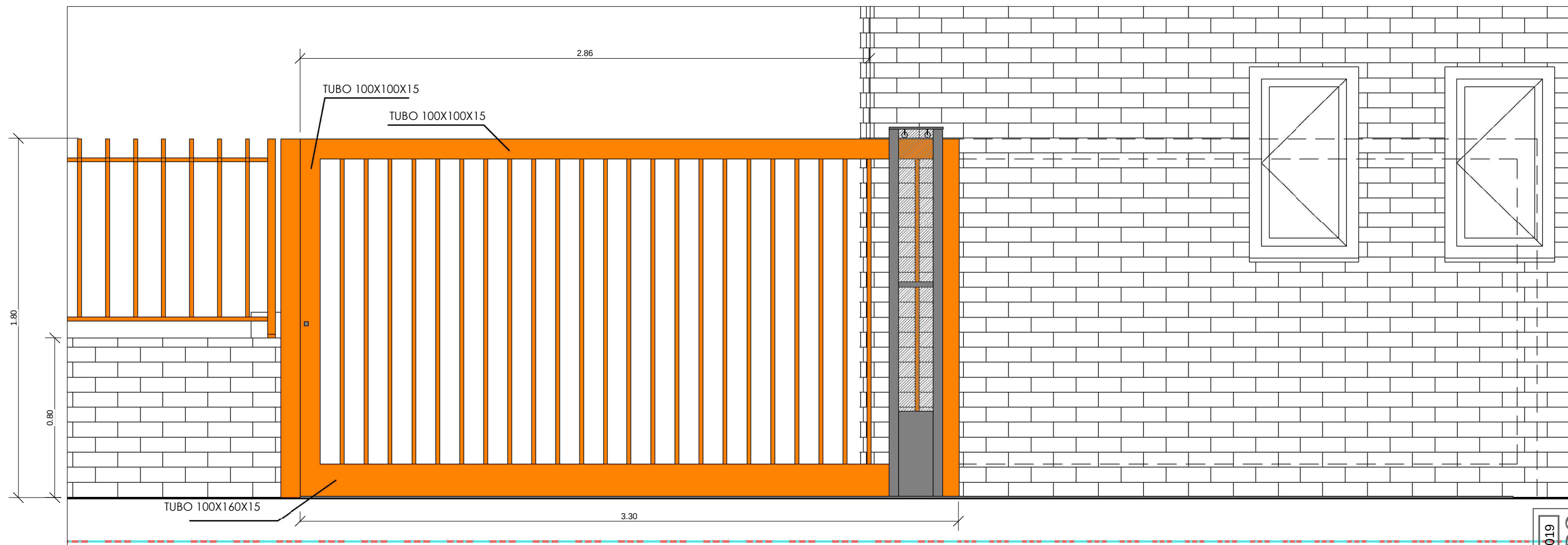
PUERTA CORREDERA 1 : 20
