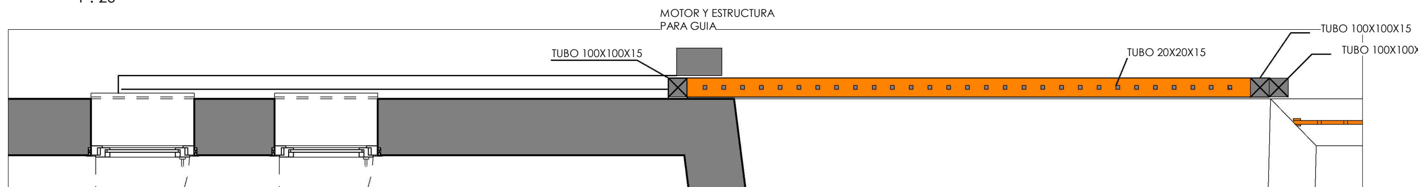
PUERTA CORREDERA 1 : 20
