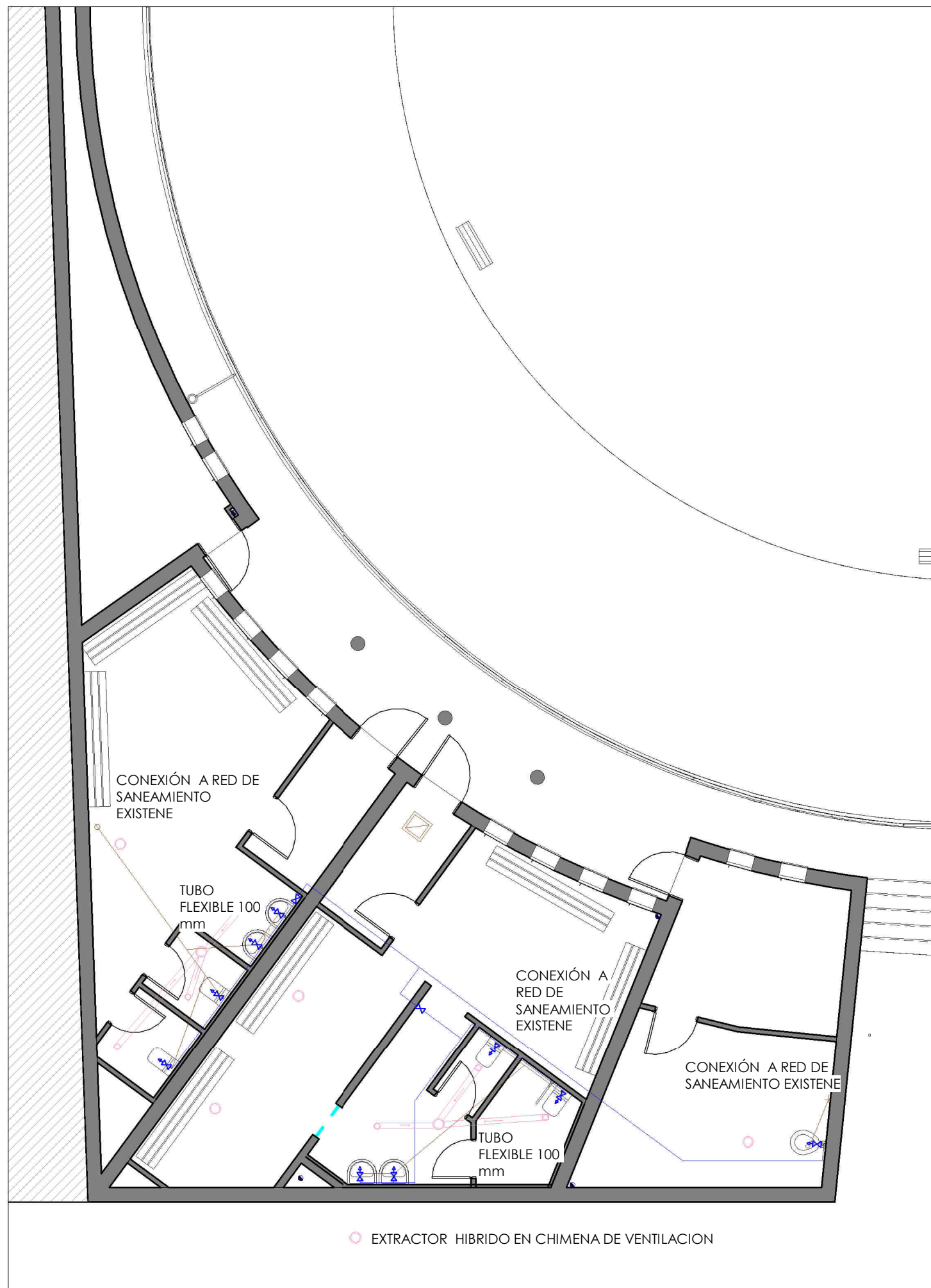
IF., VESTUARIOS 1 : 100
