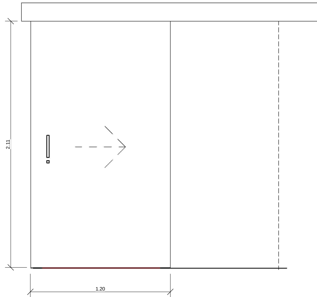
PC120 1 UD ENTRE ALMACENES PUERTA DE FORMICA CON HERRAJES DE ACERO INOX RANURA INFERIOR 1 cm PARA VENTILACIÓN
