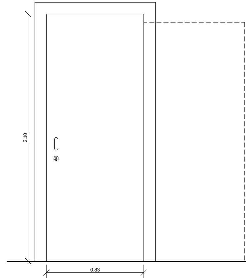
PC80 1 UD DENTRO DE BAÑO PUERTA DE FORMICA CON HERRAJES DE ACERO INOX RANURA INFERIOR 1 cm PARA VENTILACIÓN
