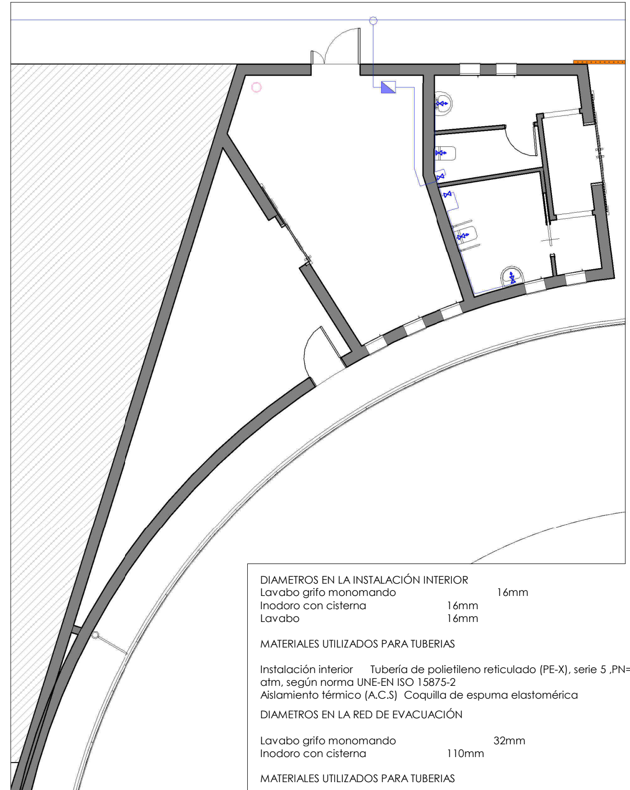
IF. BAÑOS PÚBLICOS 1 : 100
