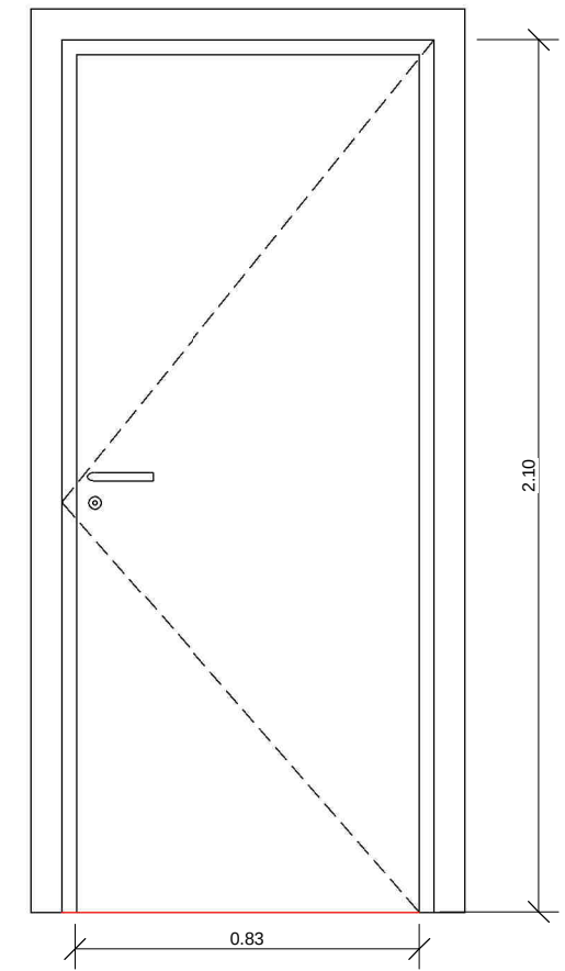
P80 8 UD DENTRO DE BAÑOS Y PUERTA ACCESO VESTUARIOS PUERTA DE FORMICA CON HERRAJES DE ACERO INOX RANURA INFERIOR 1 cm PARA VENTILACIÓN
