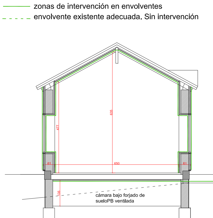
SECCIÓN TRANSVERSAL EDIFICIOS LATERALES. e:1/100
