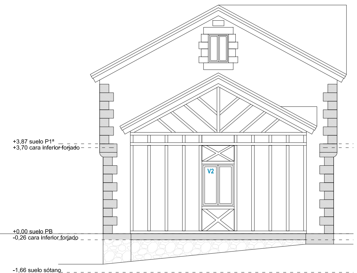
ALZADOS LATERALES . NORTE y SUR. e:1/100
