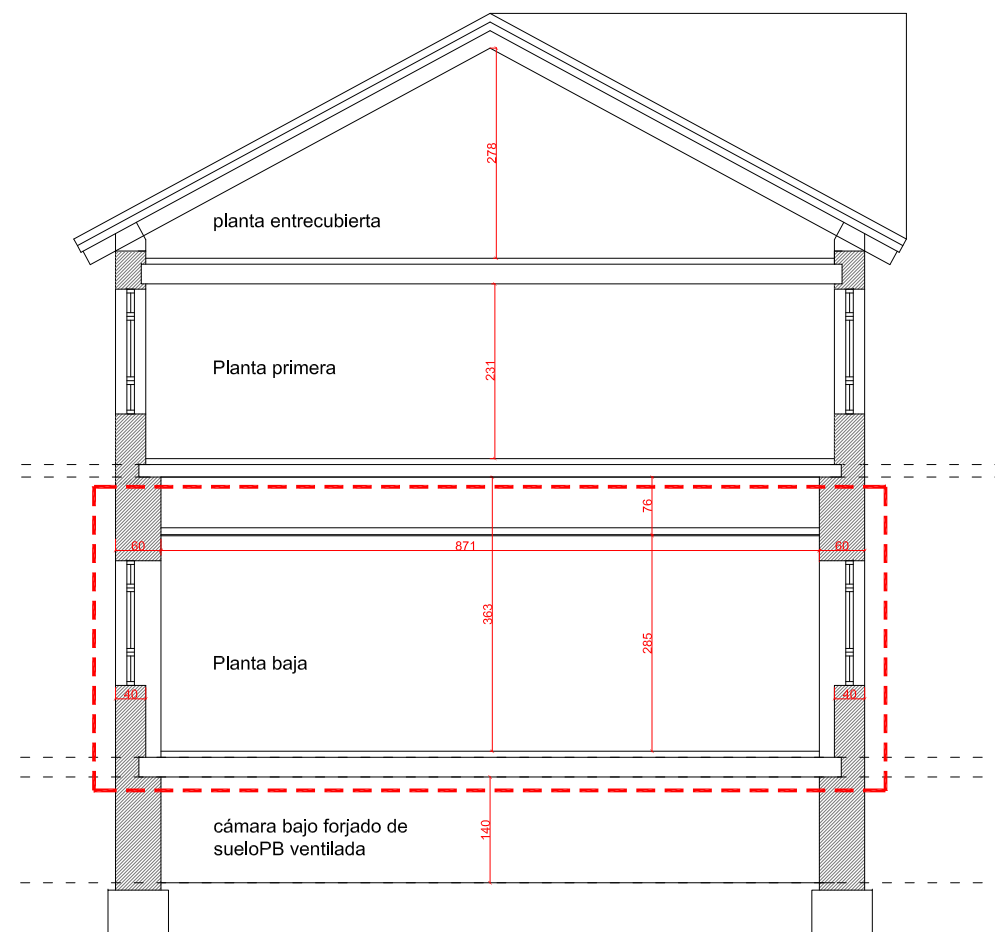
SECCIÓN TRANSVERSAL EDIFICIO CENTRAL. e:1/100
