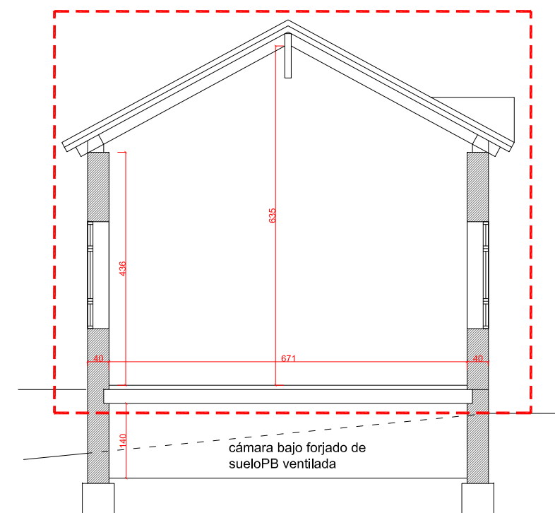
SECCIÓN TRANSVERSAL EDIFICIOS LATERALES. e:1/100
