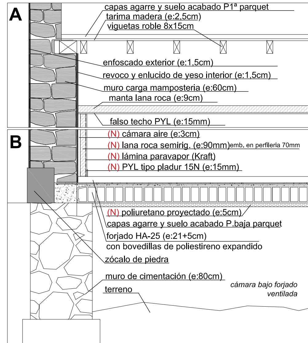
ENVOLVENTE PROPUESTA EDIFICIO CENTRAL EN PLANTA BAJA. e:1/30 (N) Nuevas capas de la envolvente propuestas. Resto de capas existentes.
