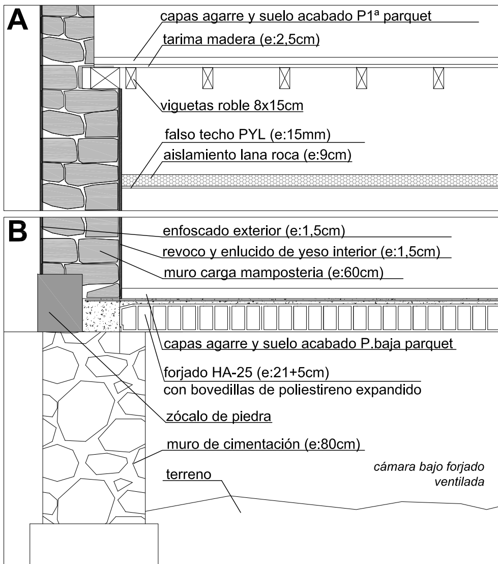
ENVOLVENTE ACTUAL EDIFICIO CENTRAL EN PLANTA BAJA. e:1/30
