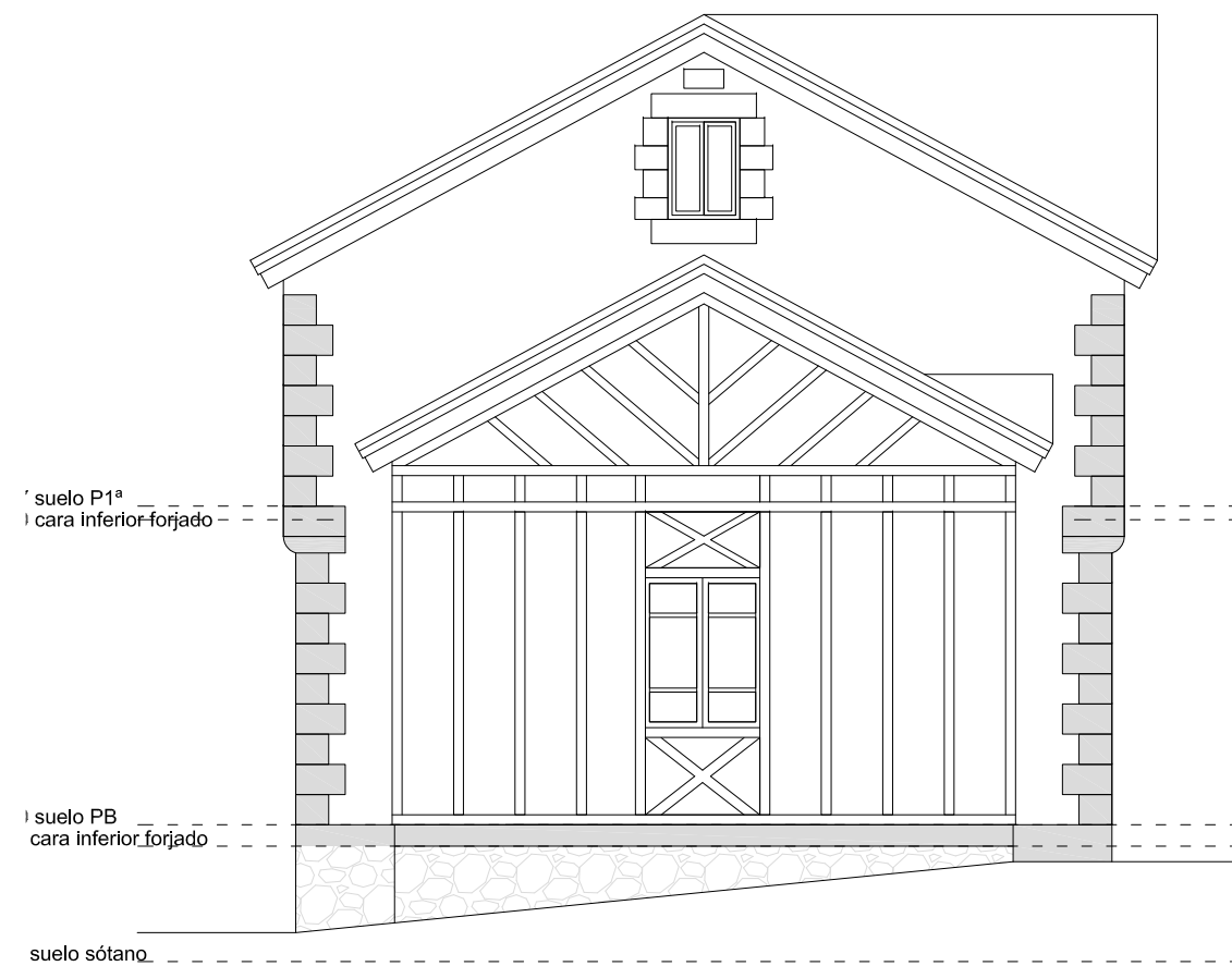
ALZADOS LATERALES . NORTE y SUR. e:1/100
