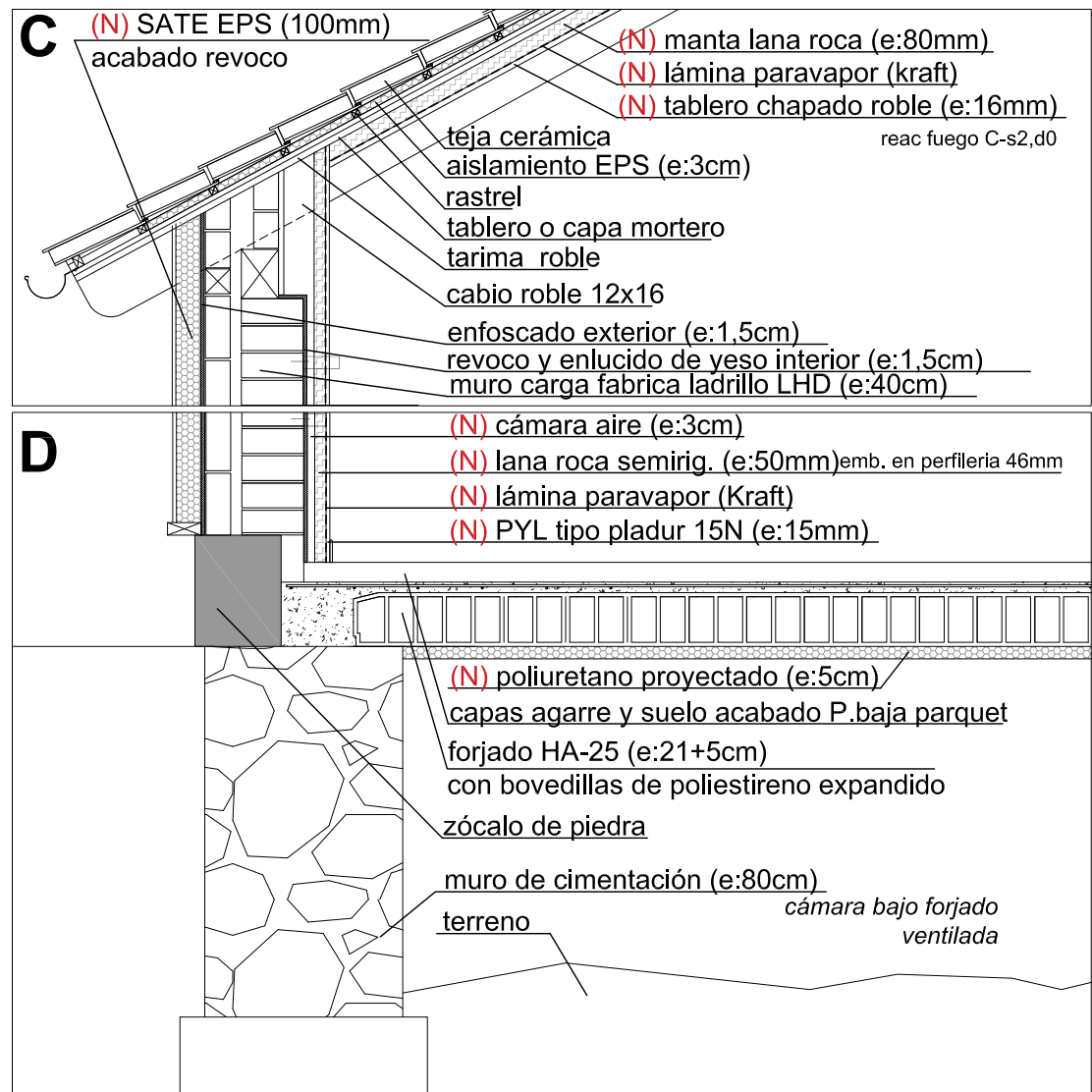
ENVOLVENTE PROPUESTA EDIFICIOS LATERALES. e:1/30
