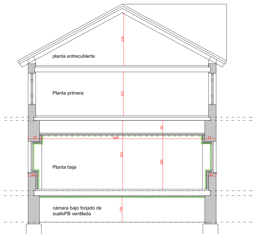
SECCIÓN TRANSVERSAL EDIFICIO CENTRAL. e:1/100
