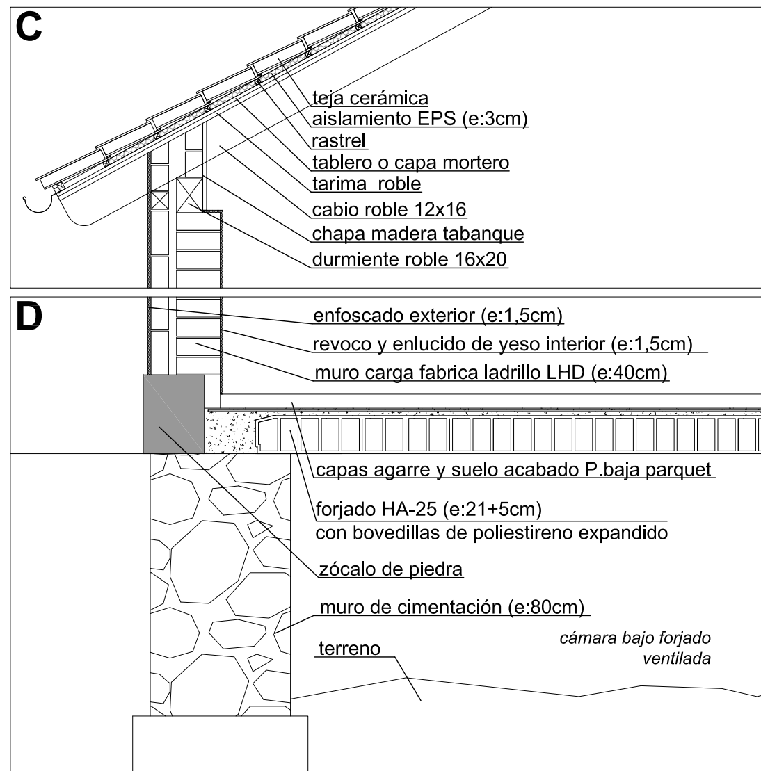
ENVOLVENTE ACTUAL EDIFICIOS LATERALES. e:1/30
