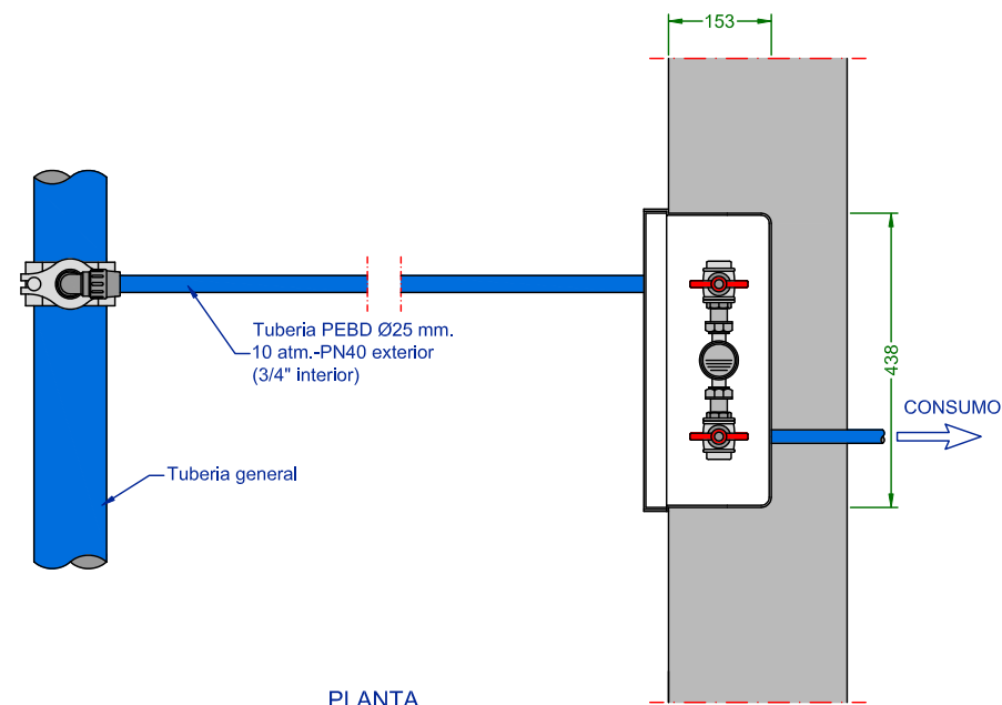
PLANTA
