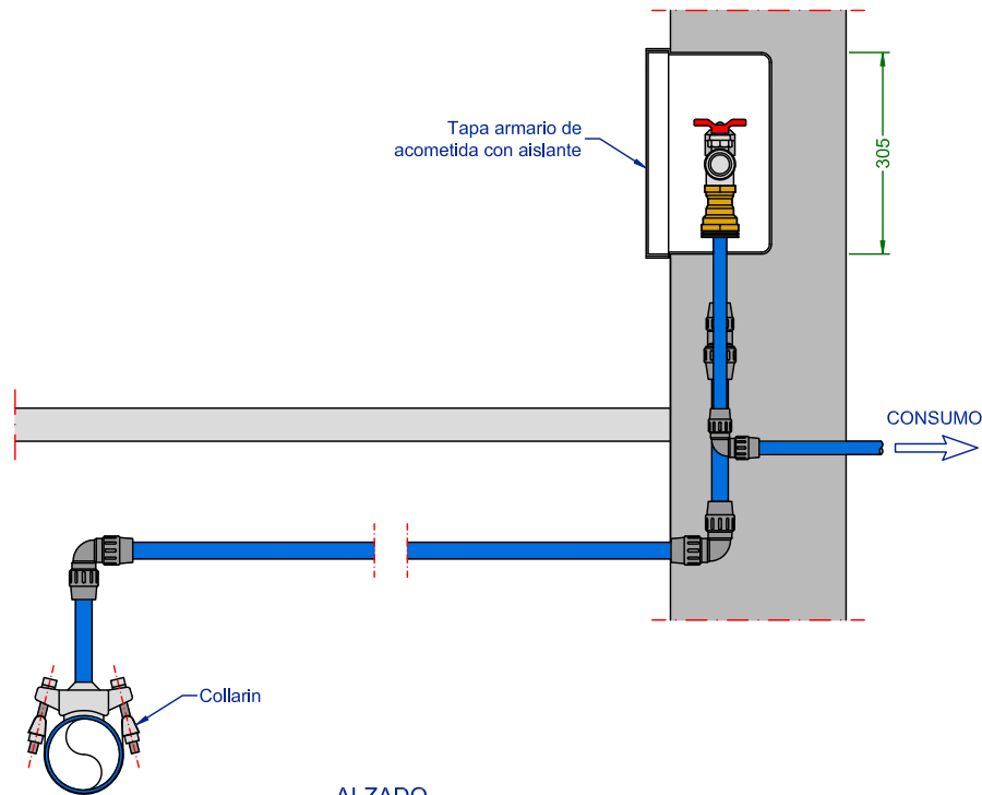
ALZADO
