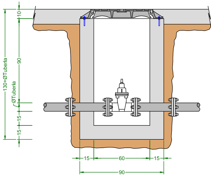
SECCION
