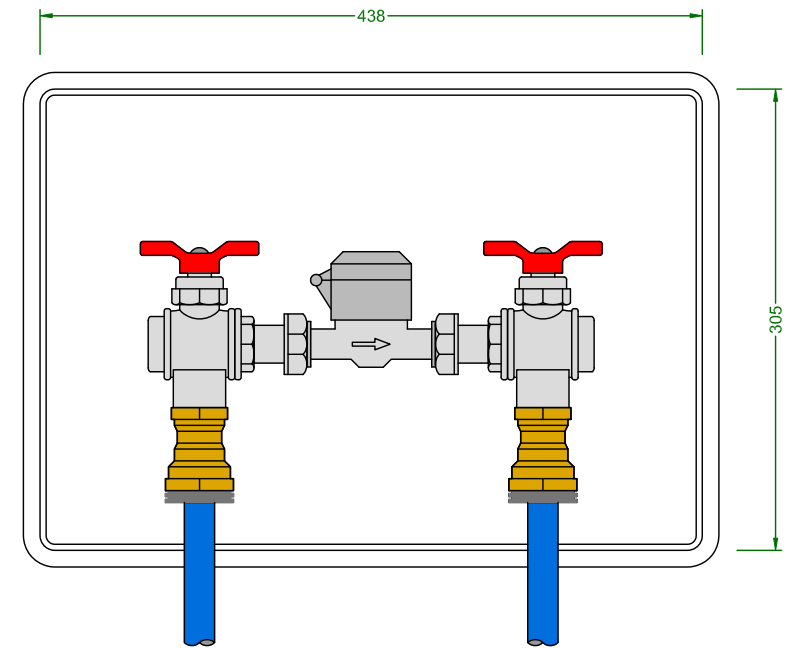
SECCION
