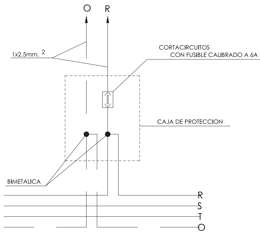
ESQUEMA DE CONEXION A LUMINARIA
