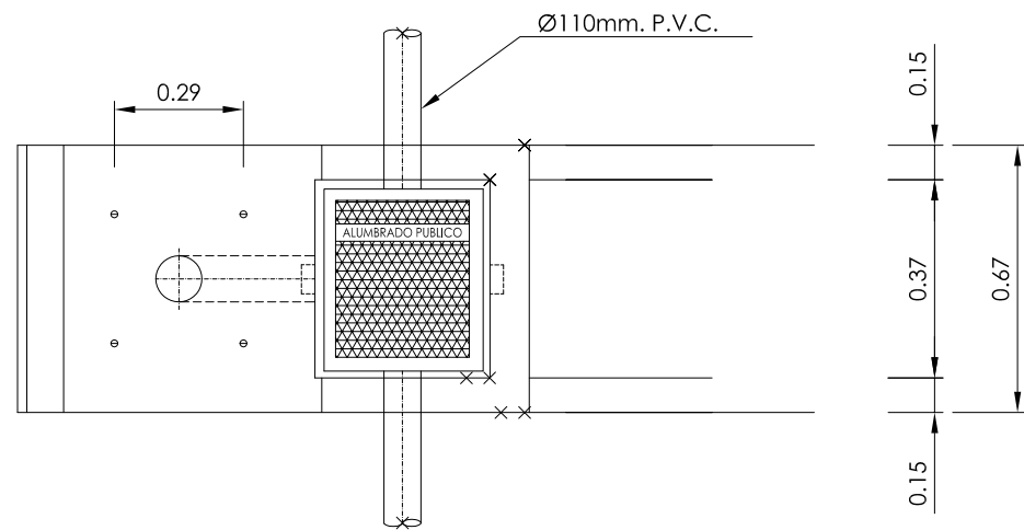
CIMENTACION DE COLUMNA CON ARQUETA ADOSADA
