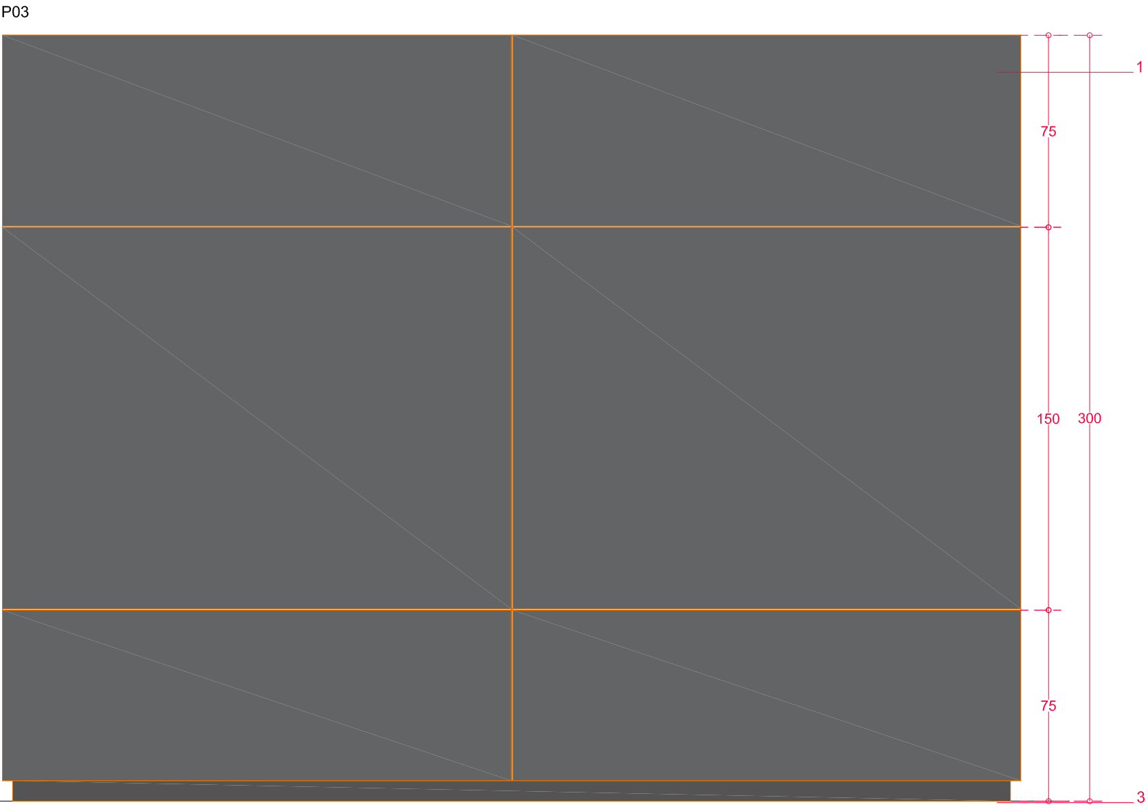
alzado frontal
