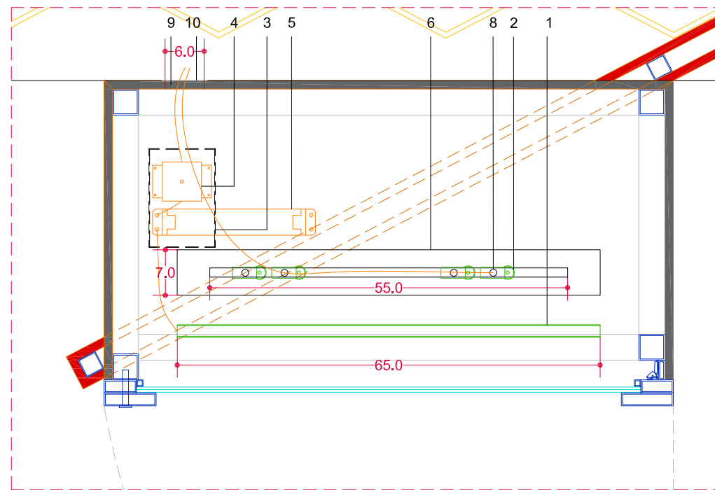
Planta Cotas en cm E 1:8
