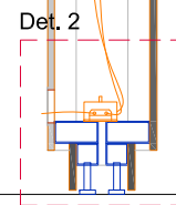
Sección Cotas en cm E 1:15
