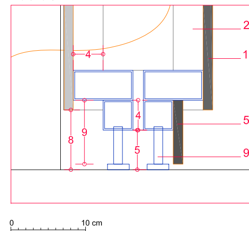
Detalle 3
