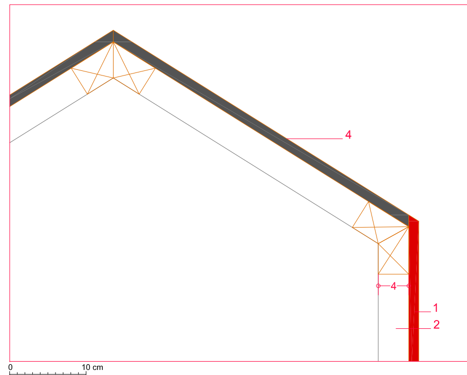
Detalle 1
