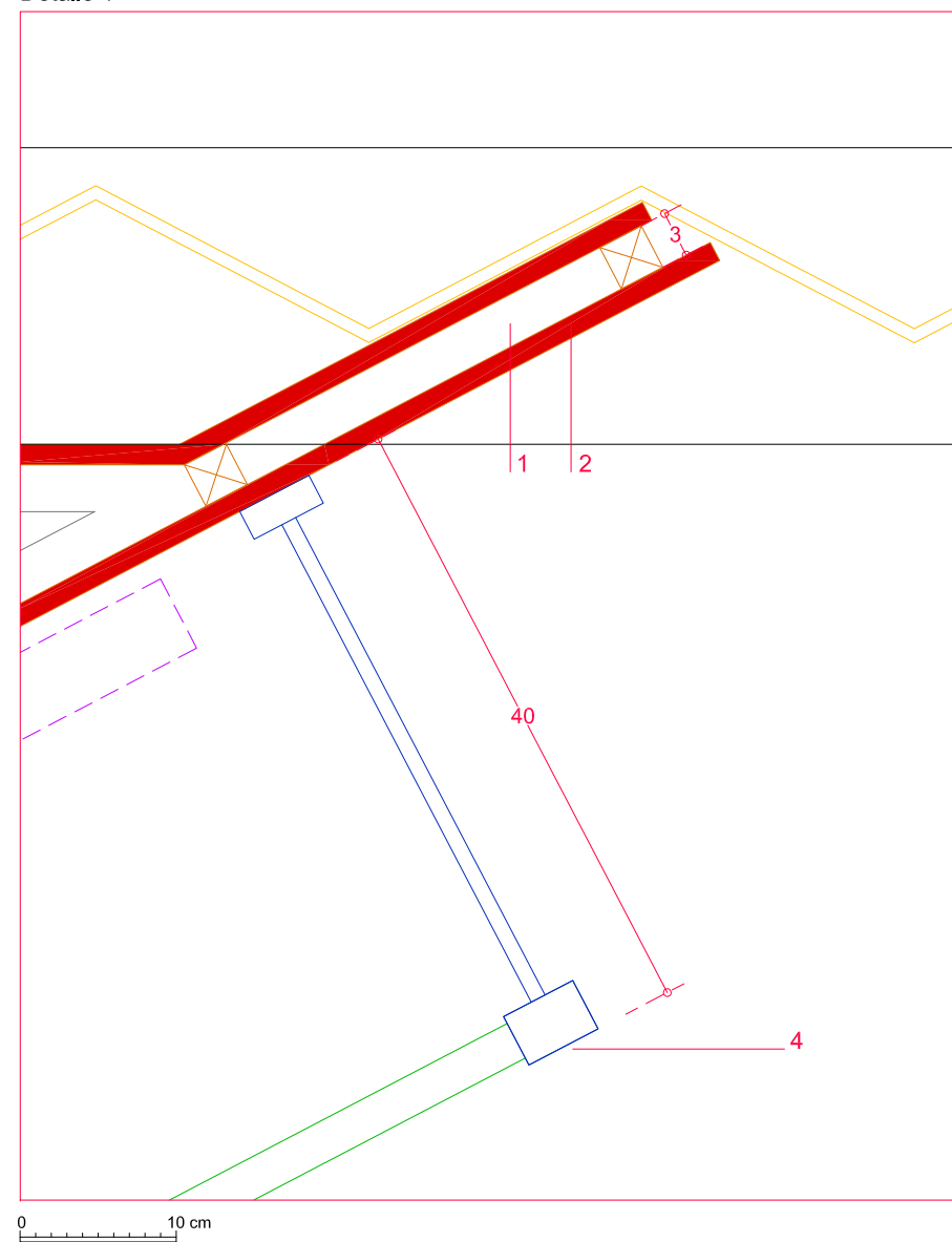
Detalle 1
