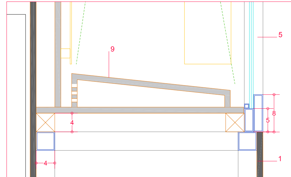
Detalle 2
