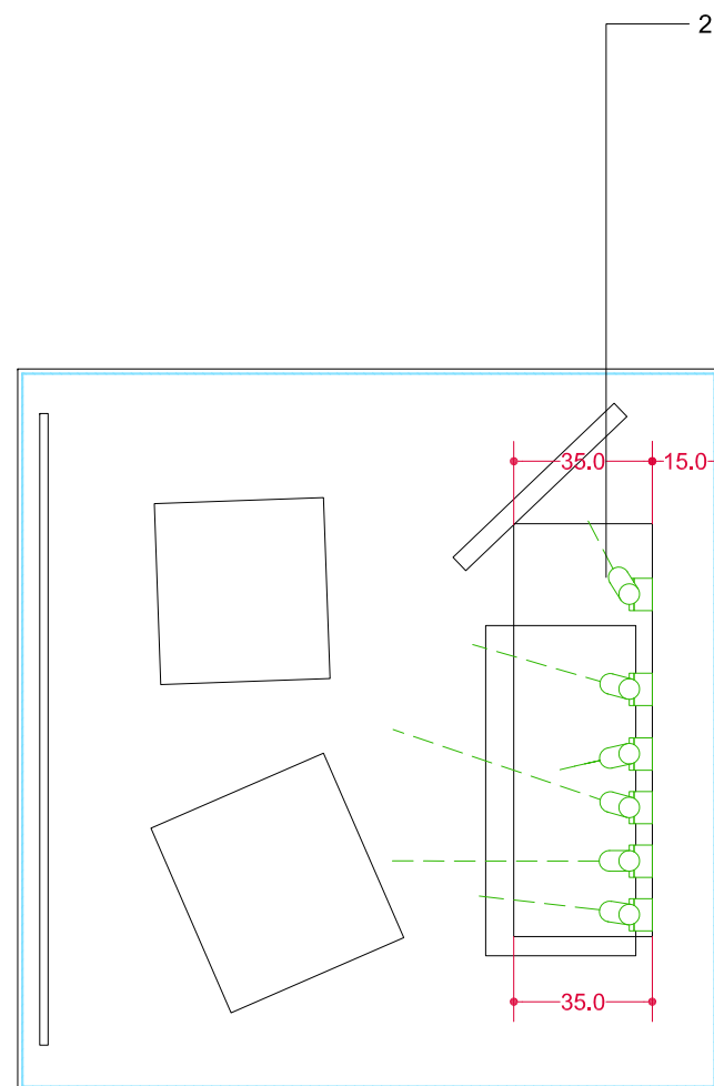
PLANTA E 1:20 Cotas en cm. (*) medida aproximada
