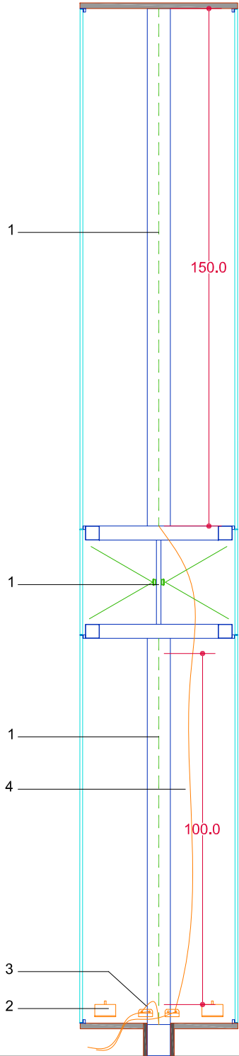
Sección Cotas en cm E 1:15
