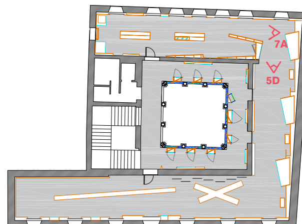
Vista nuevo murete 7A *los elementos gráficos son meramente orientativos
