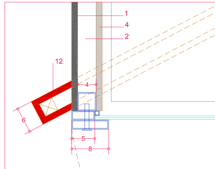
Detalle 1
