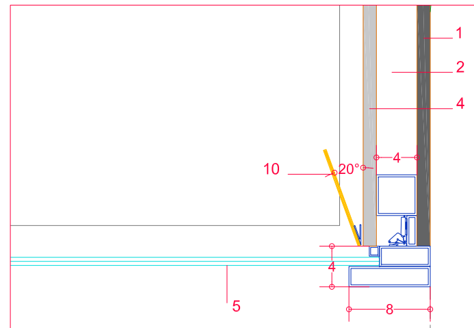
Detalle 2
