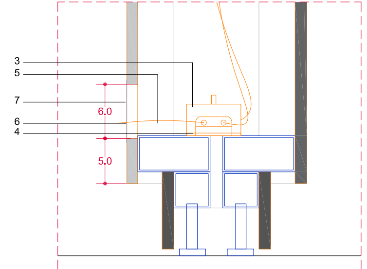
Detalle 2 E 1:4
