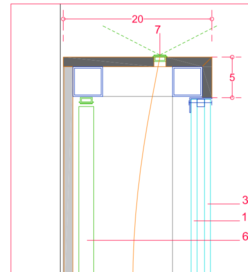
Detalle 1
