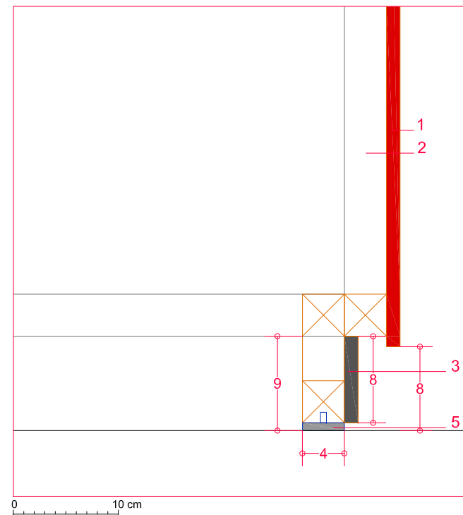
Detalle 2
