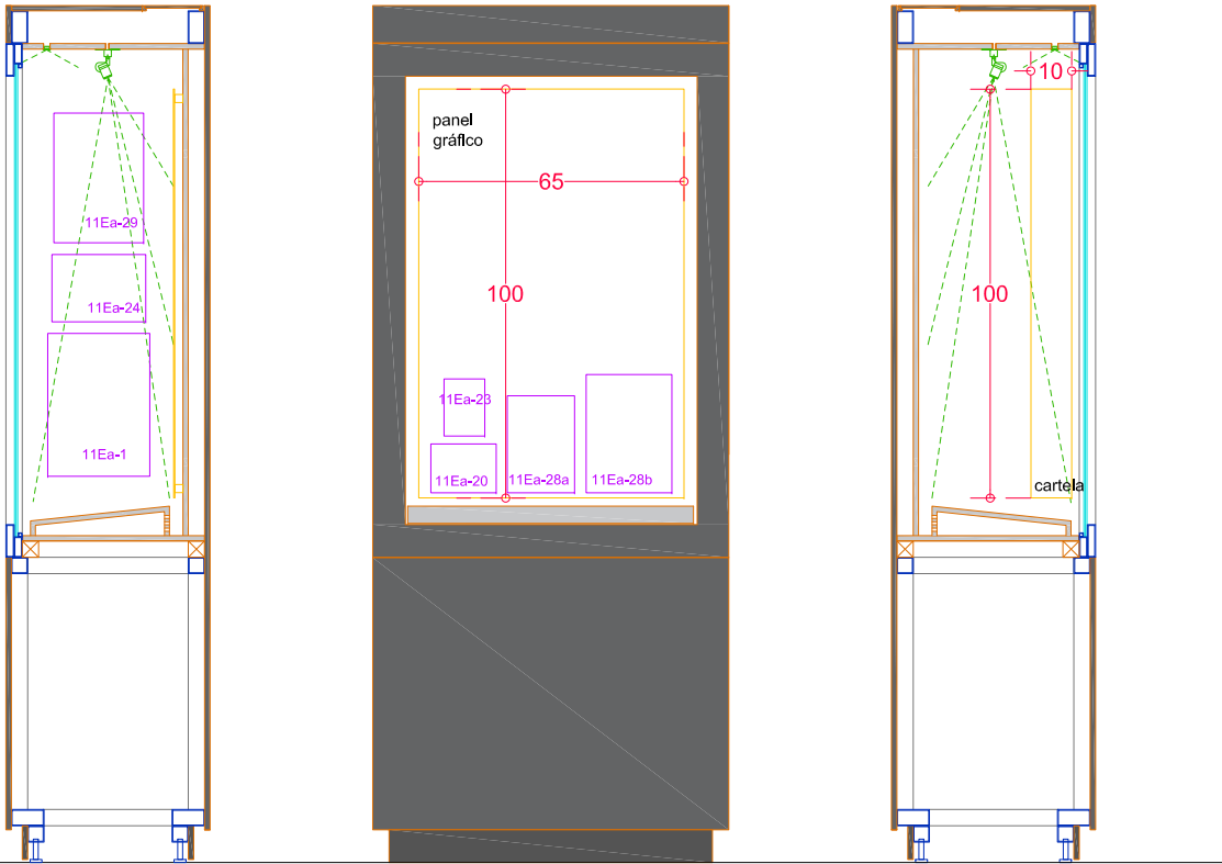
sección vertical izquierda
