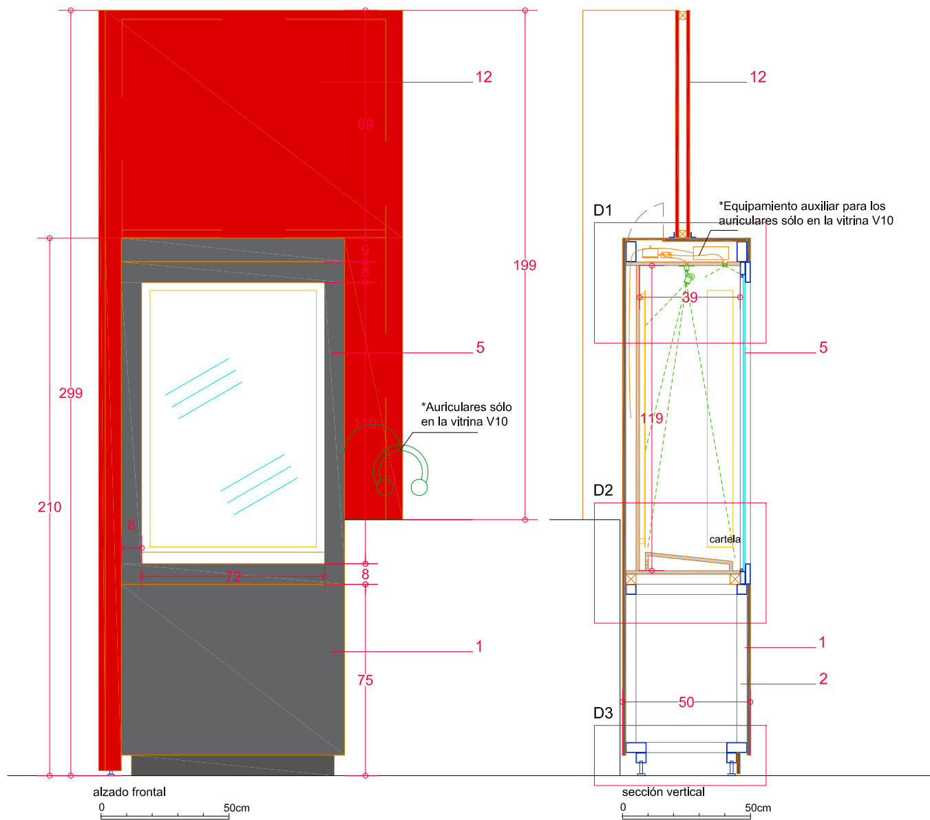
Detalle 2
