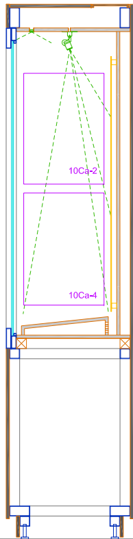
sección vertical izquierda
