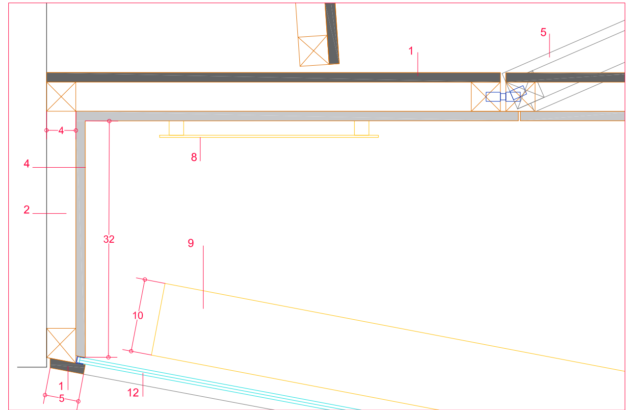
Detalle 1
