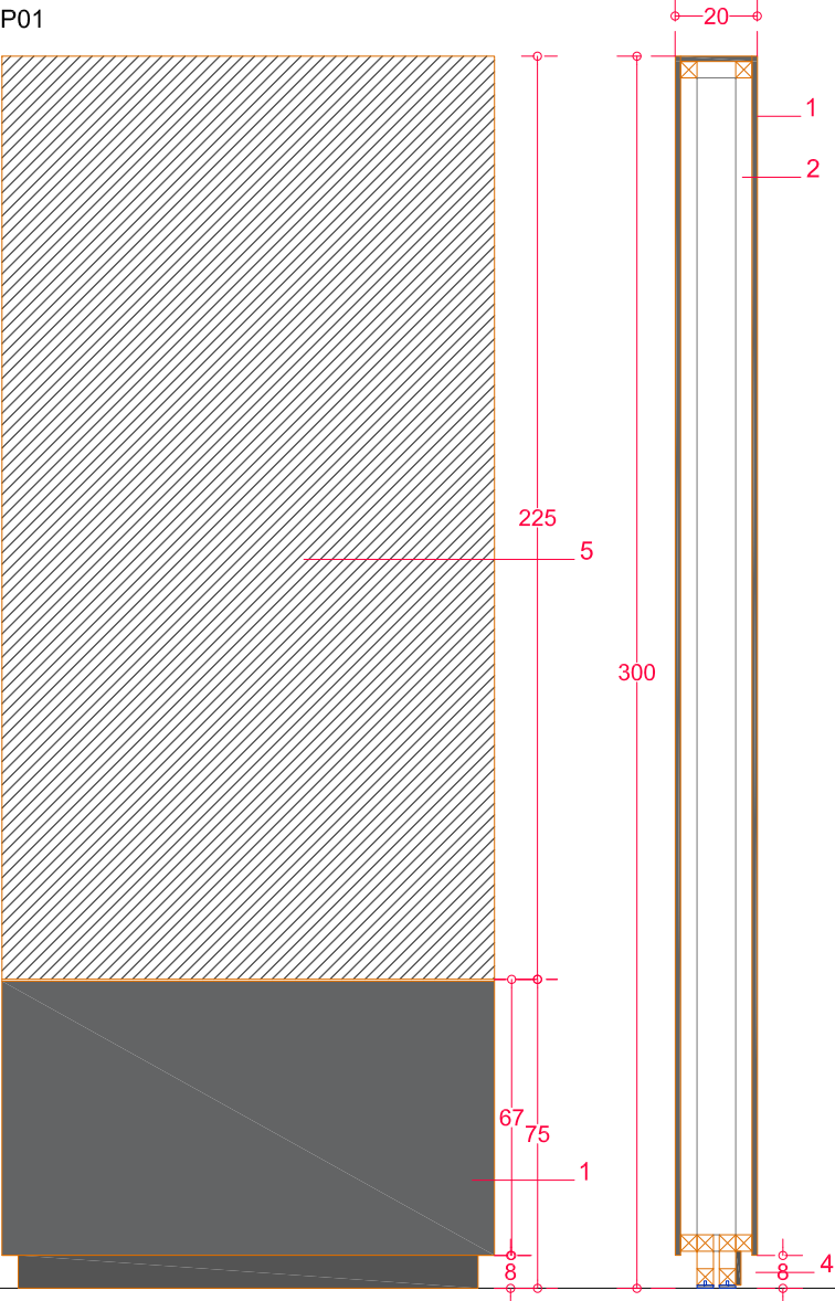
alzado frontal
