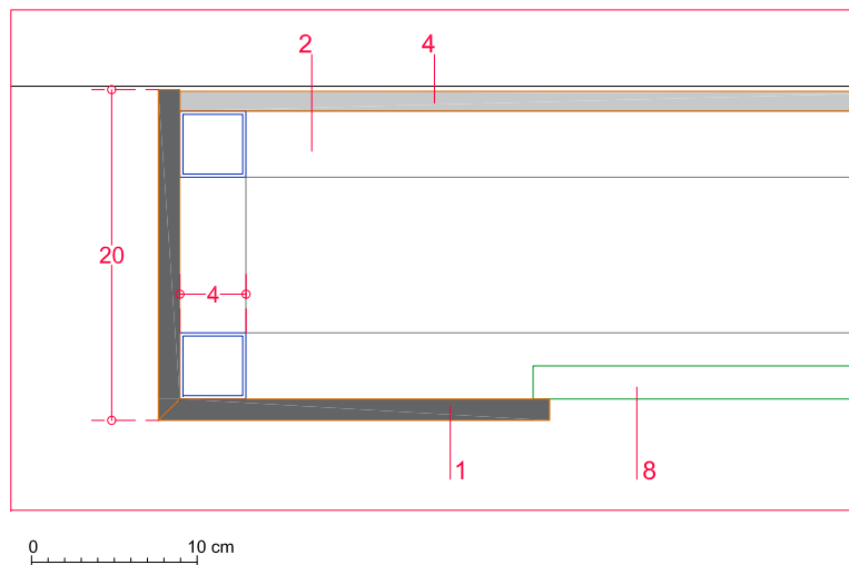
Detalle 4
