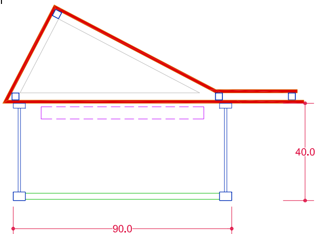
Planta Cotas en cm E 1:15
