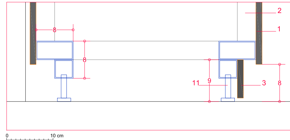
Detalle 3
