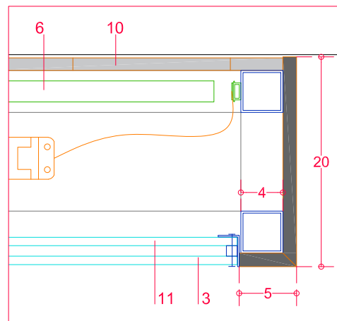
Detalle 5
