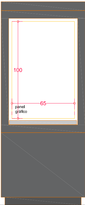
alzado frontal
