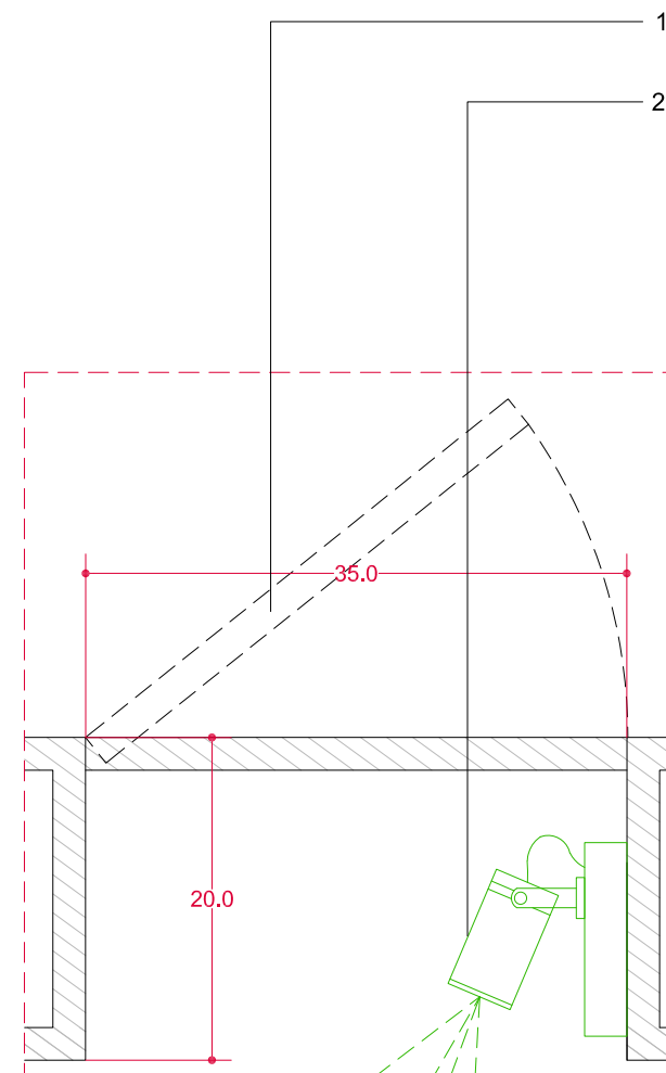
DETALLE 1 E 1:5 Cotas en cm.
