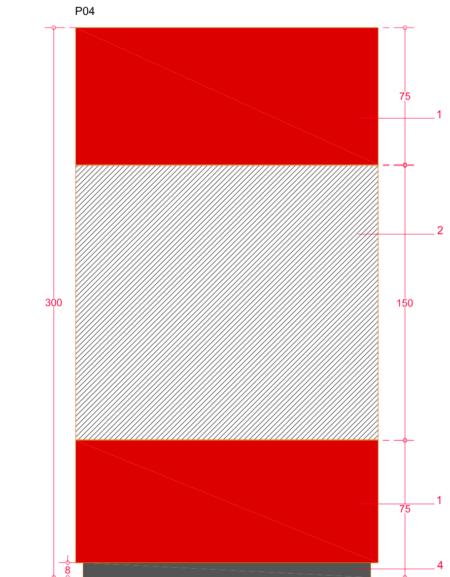
alzado frontal
