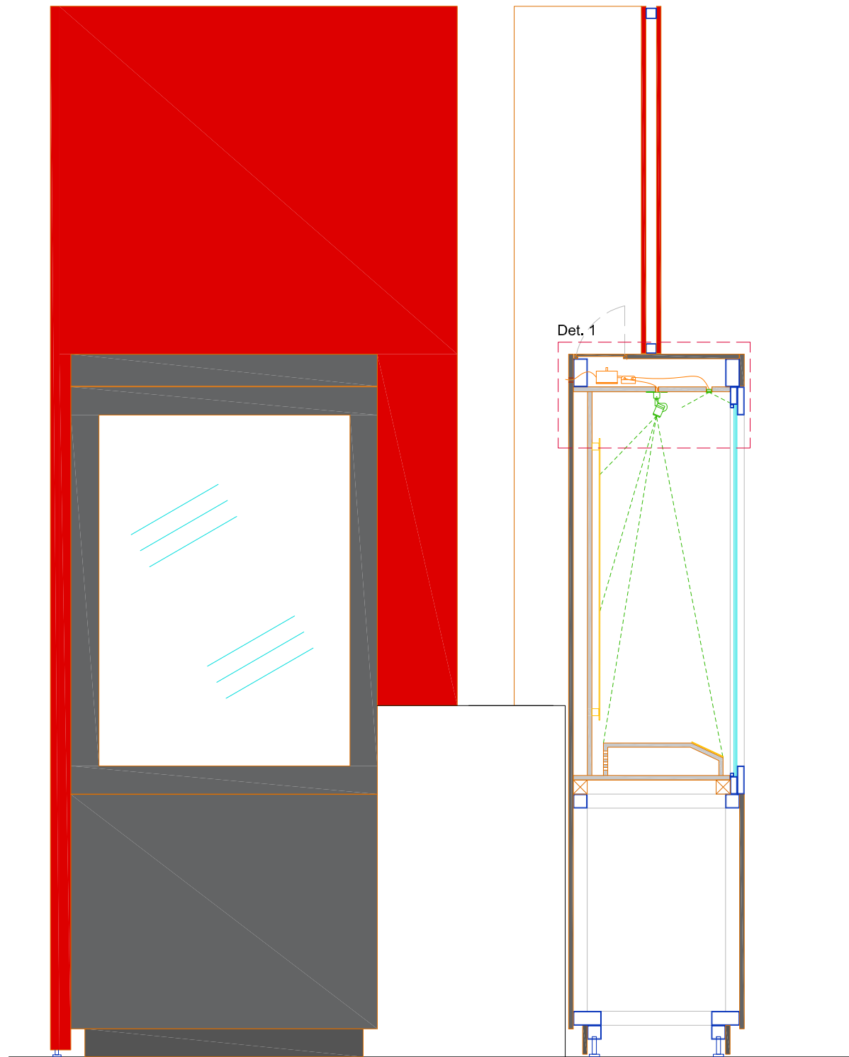
Alzado frontal Cotas en cm E 1:15
