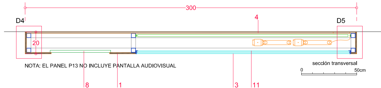
Detalle 4
