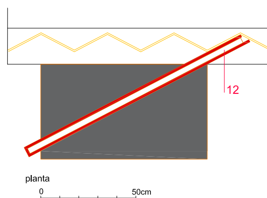
Detalle 3
