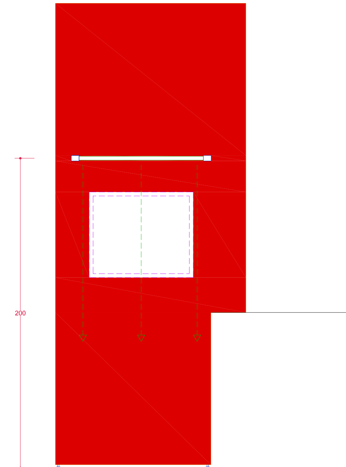
Alzado frontal Cotas en cm E 1:15
