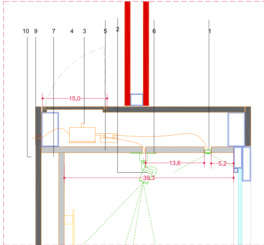
Detalle 1 Cotas en cm E 1:5
