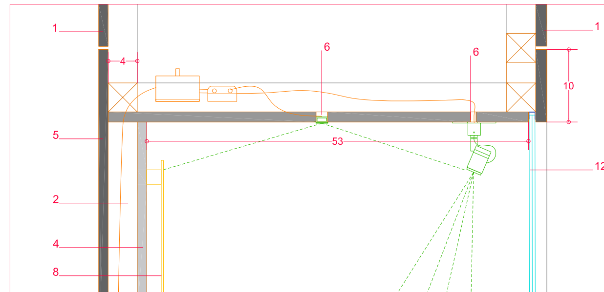
Detalle 1
