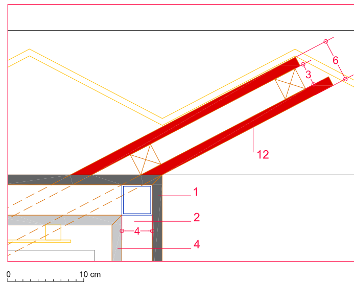
Detalle 3
