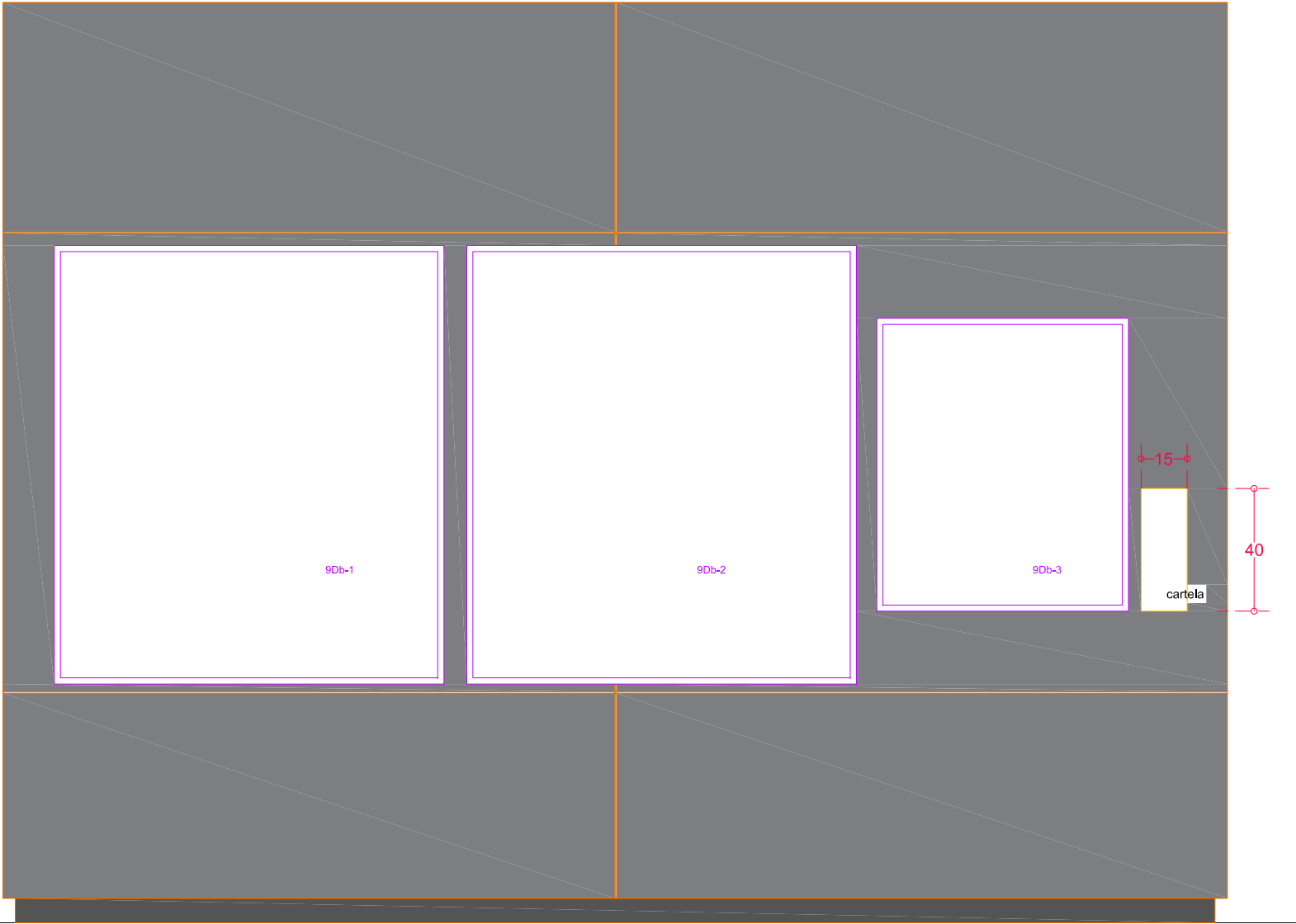
alzado frontal
