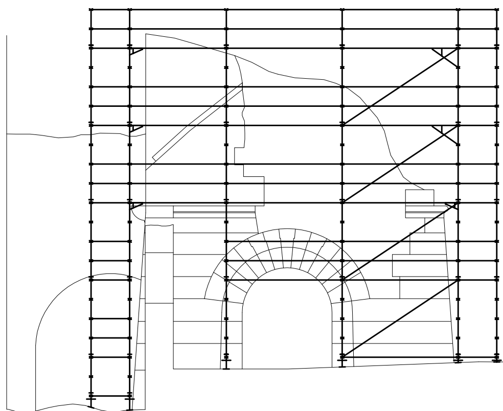
ALZADO ESTE
