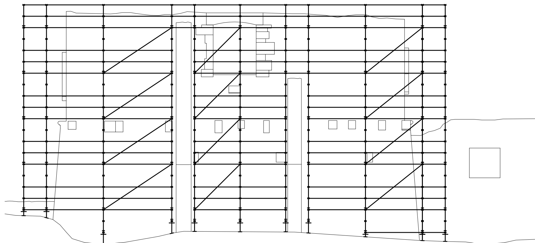
ALZADO SUR
