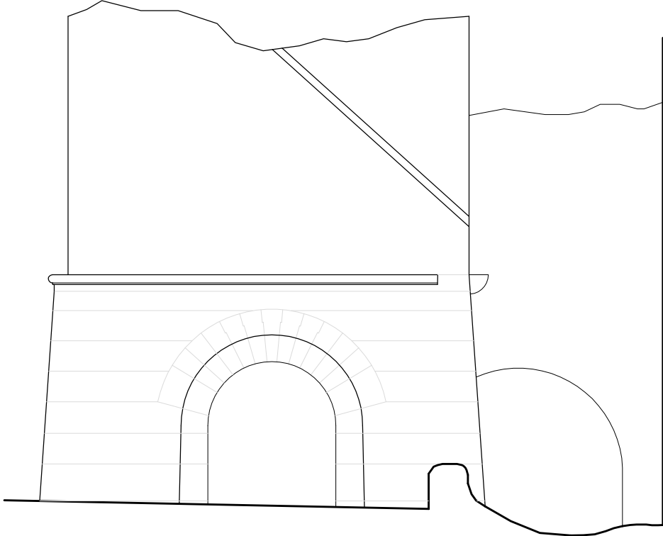
ALZADO OESTE
