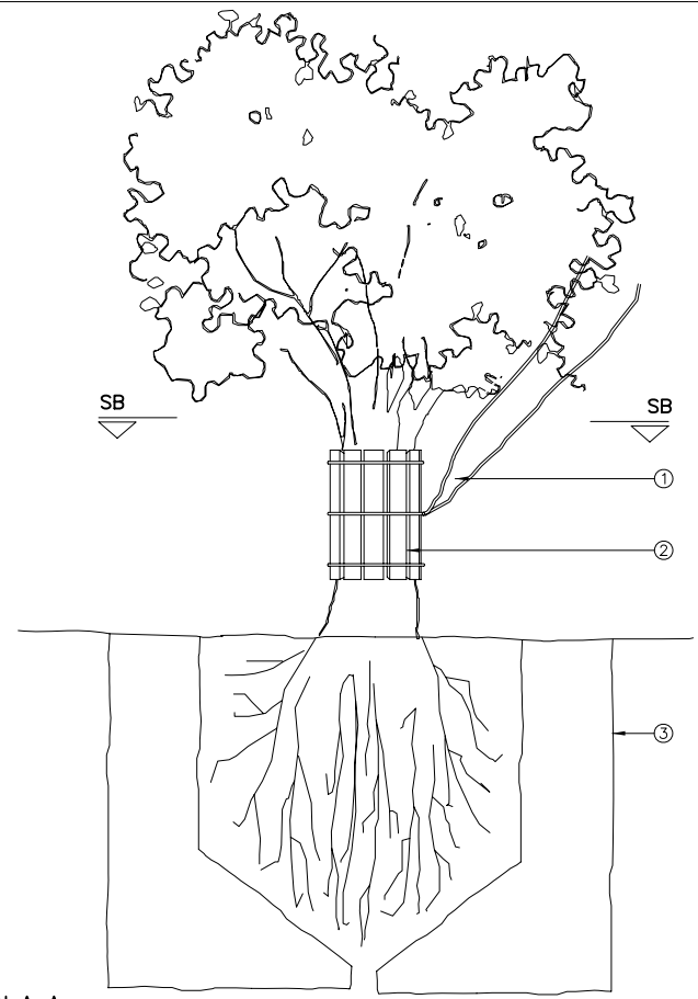
SECCIÓN A-A
