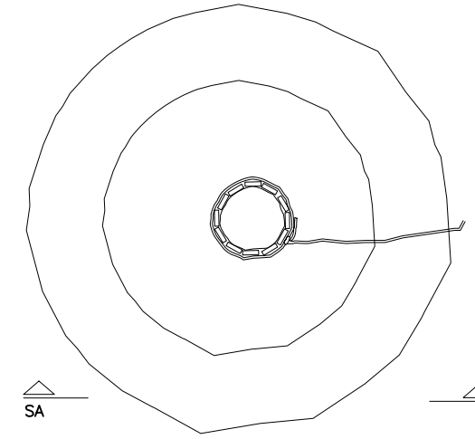
SECCIÓN B-B
