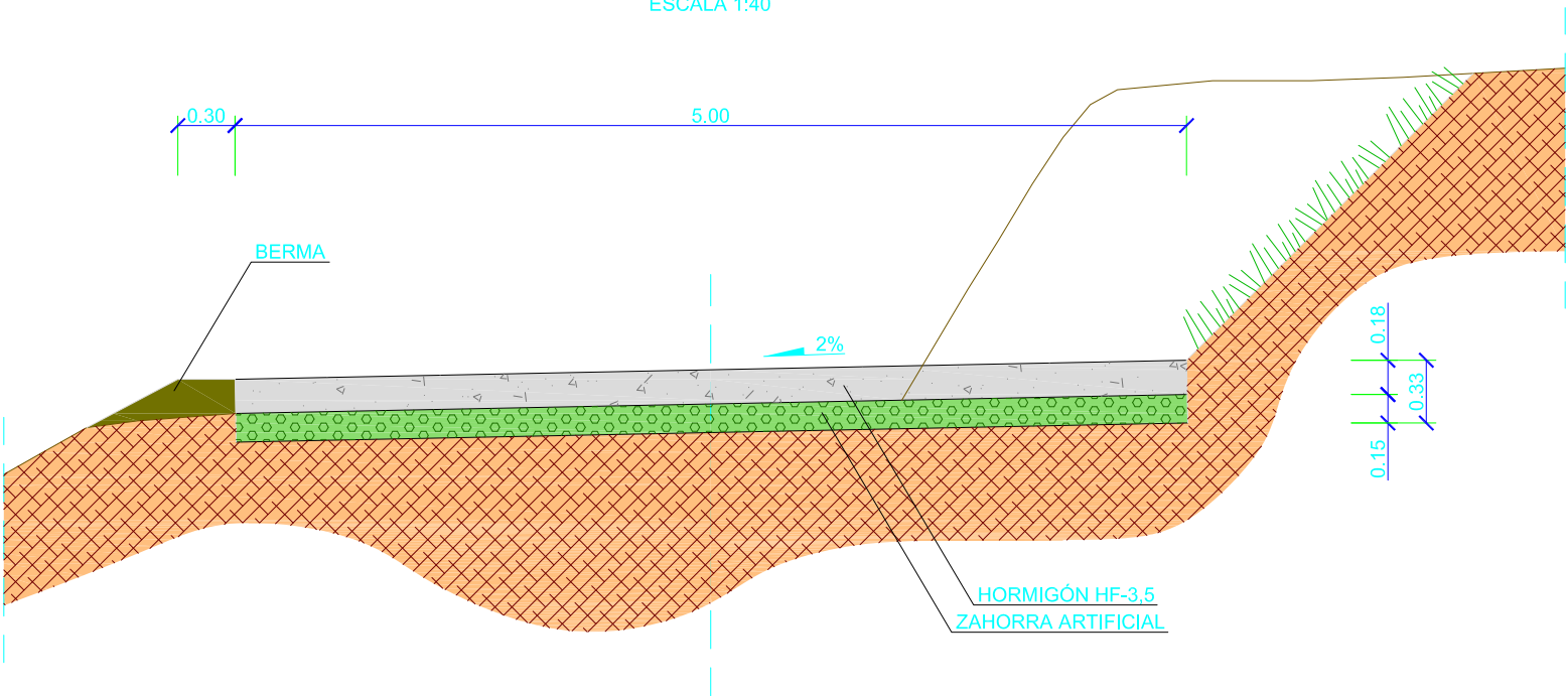
SECCIÓN TIPO 0+080 ESCALA 1:40
