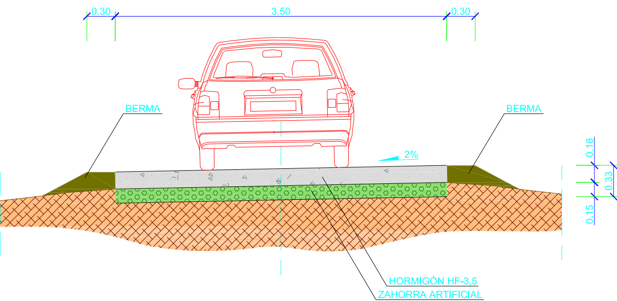
SECCIÓN TIPO 0+100 ESCALA 1:40
