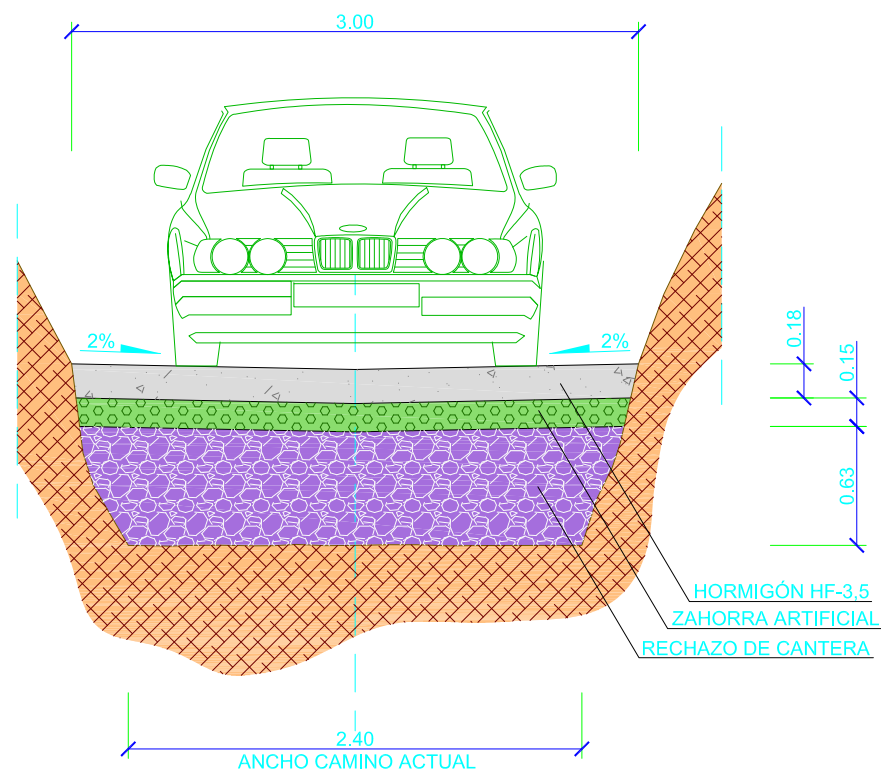
SECCIÓN TIPO 0+030 ESCALA 1:40
