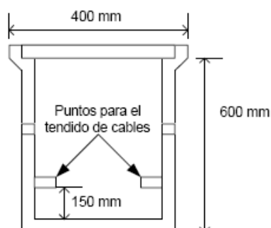
Alzado frontal
