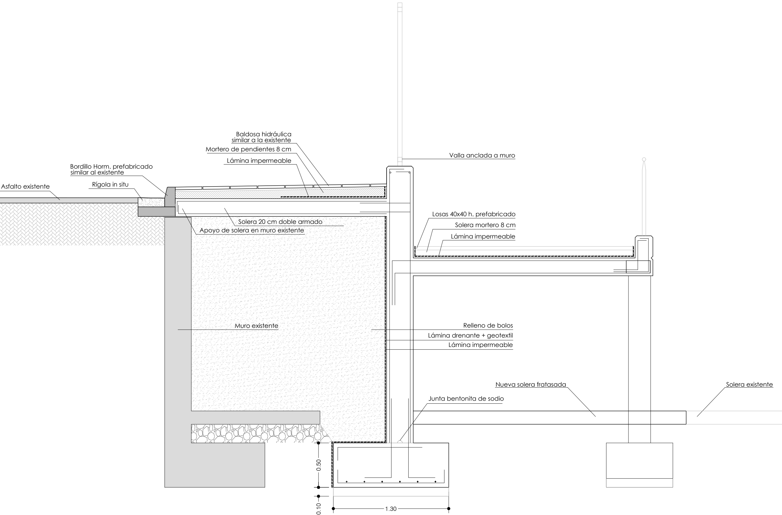
DETALLE CONSTRUCTIVO e 1/25
