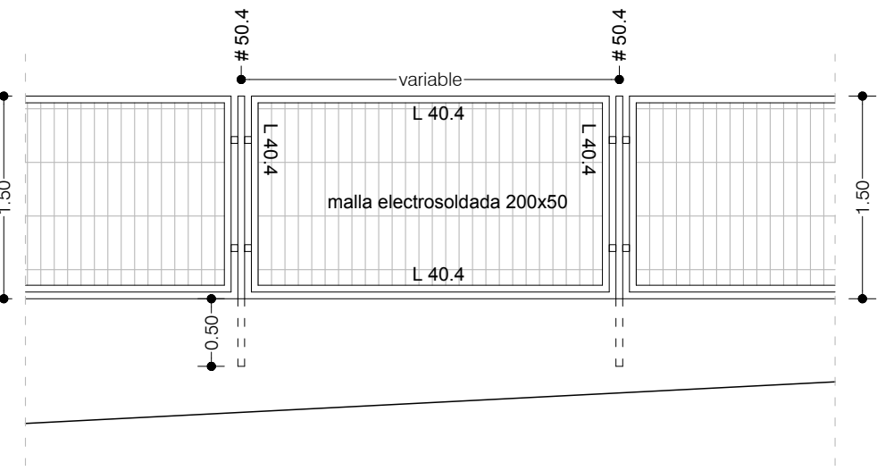
V1 Valla de cierre Lacado en color a elegir por la DF
