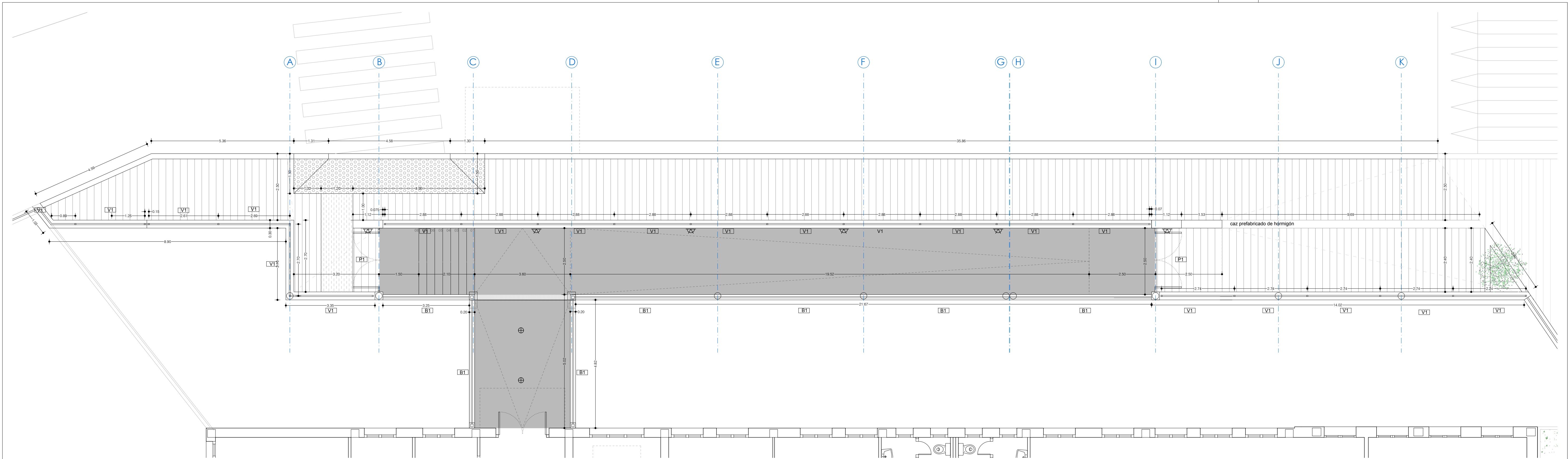
PLANTA DE LA INTERVENCIÓN e 1/75
