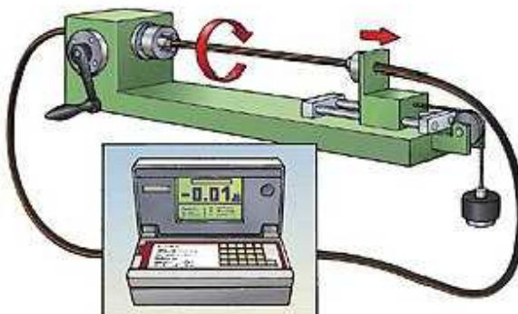
Figura 20.- Ejecución de la prueba según EN 187000 Método 508.
