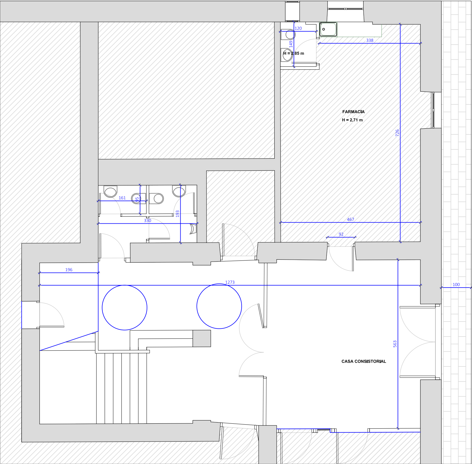
PLANTA ACOTADA
