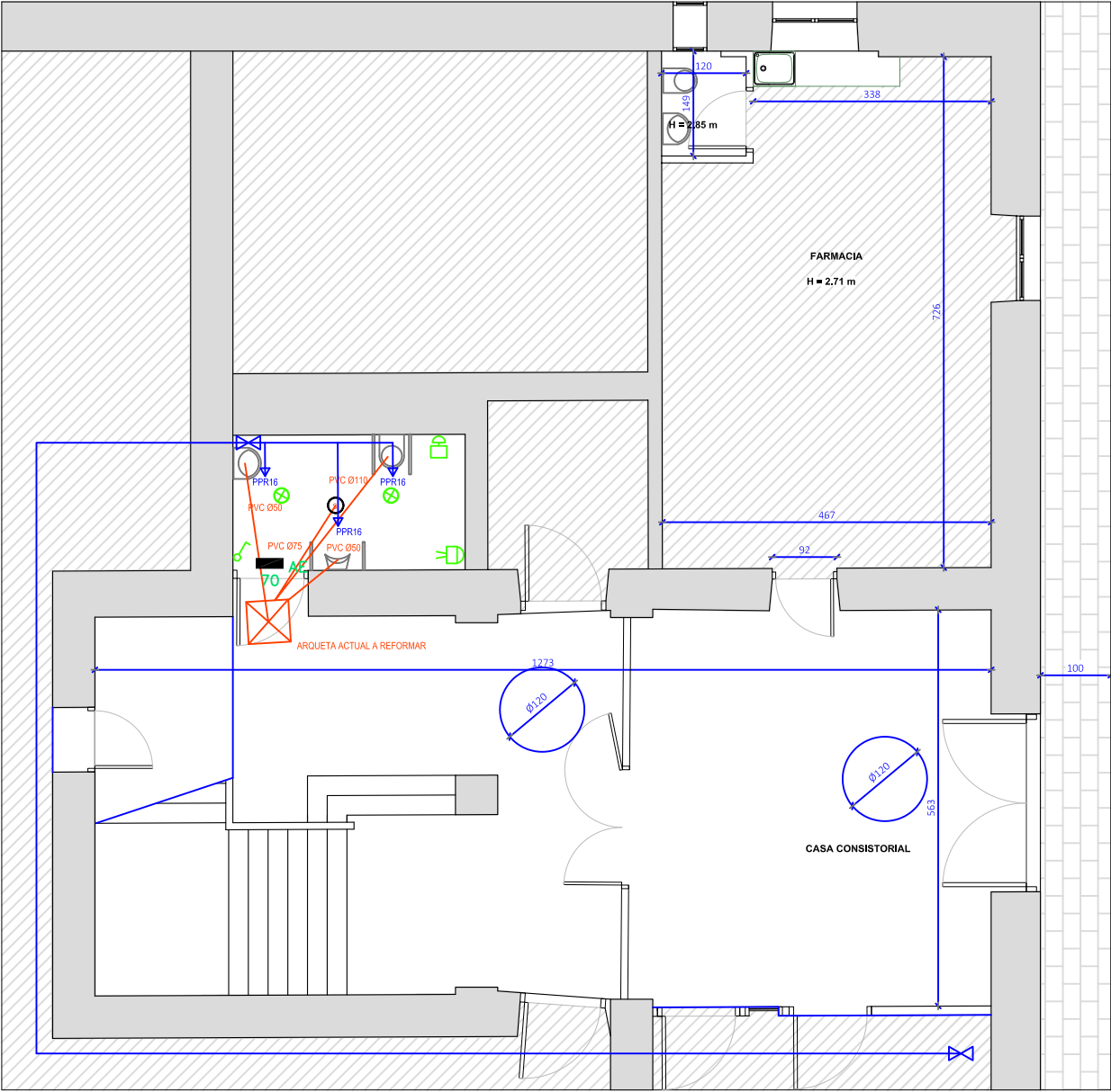
PLANTA INSTALACIONES
