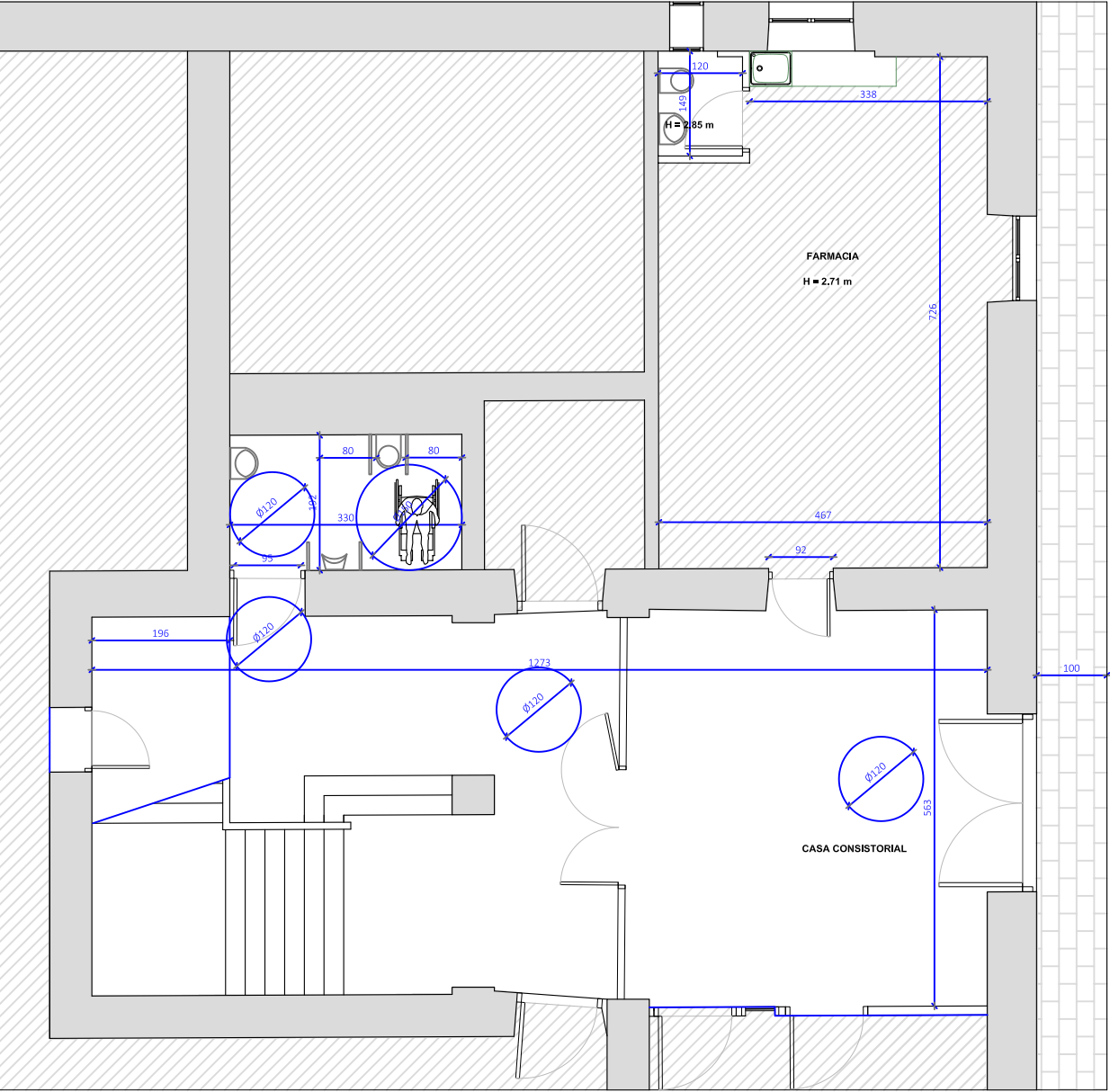
PLANTA ACOTADA
