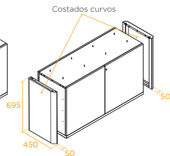
MÓDULO INDEPENDIENTE
