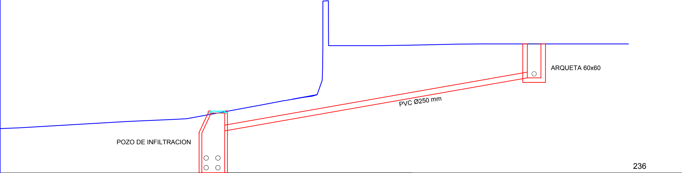
SECCION TRANSVERSAL E. 1:100
