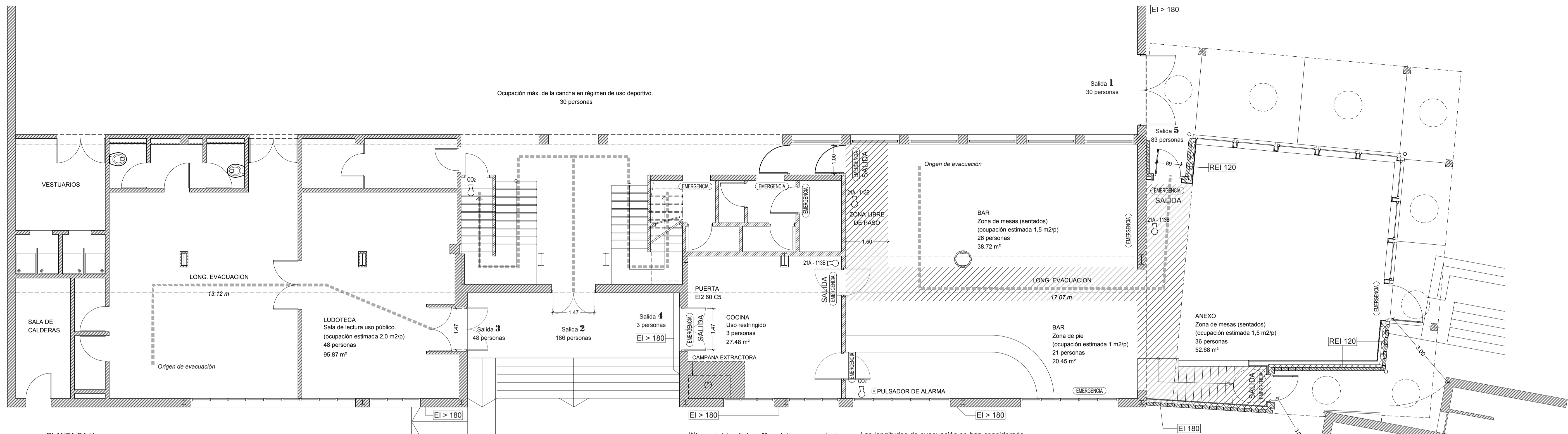
PLANTA BAJA E: 175
