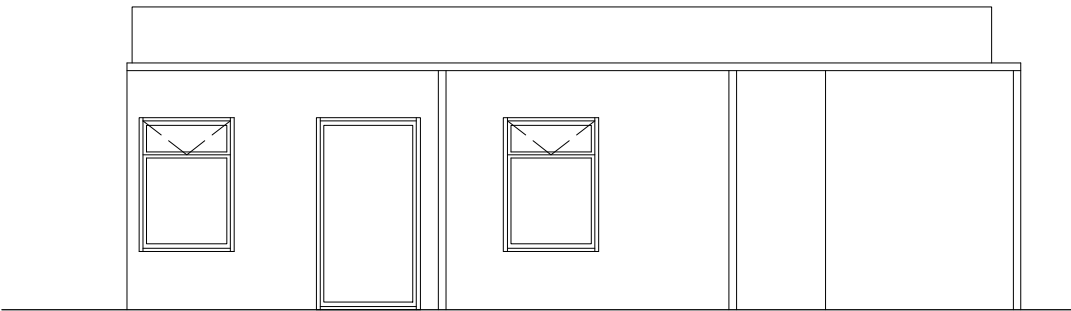
ALZADO 1 PATIO
