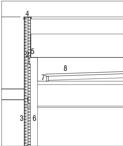
SECCION LONGITUDINAL
