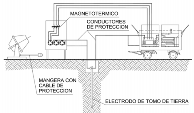
INTERRUPTOR AUTOMATICO
