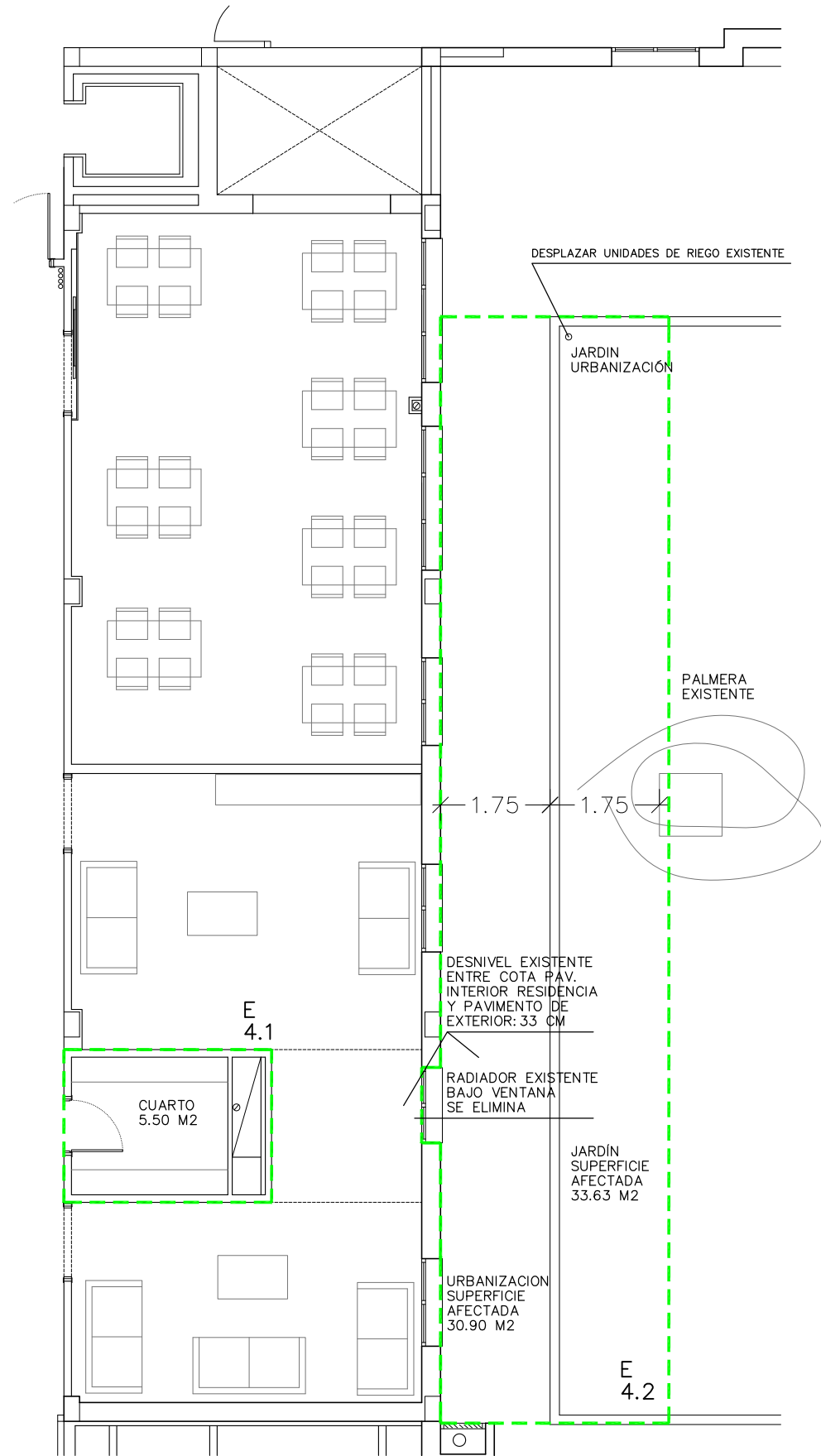
ESTADO ACTUAL DISTRIBUCIÓN SUPERFICIES AMBITO DE ACTUACIÓN
