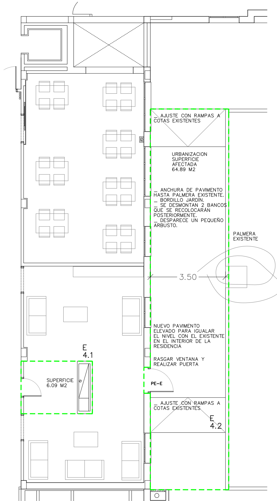
ESTADO FUTURO DISTRIBUCIÓN SUPERFICIES AMBITO DE ACTUACIÓN
