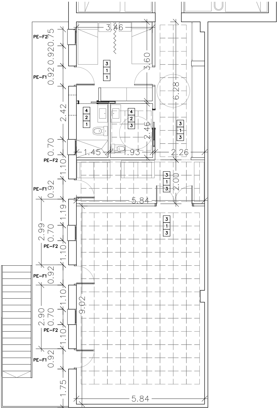
ACOTACIÓN FALSOS TECHOS ACABADOS Y ALTURAS
