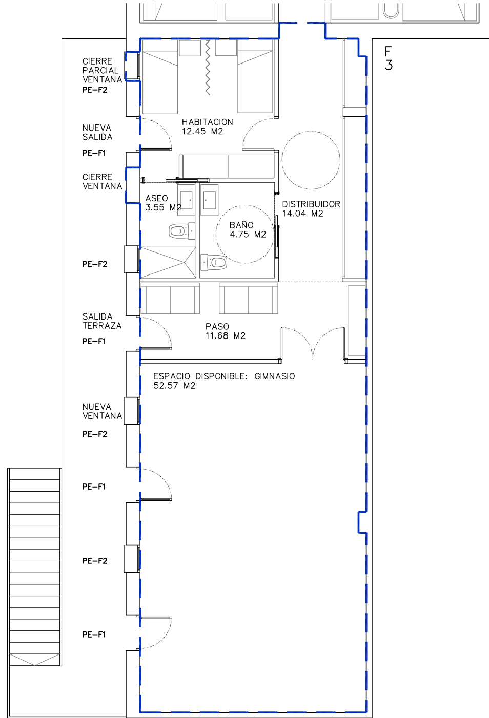
ESTADO FUTURO DISTRIBUCIÓN SUPERFICIES AMBITO DE ACTUACIÓN
