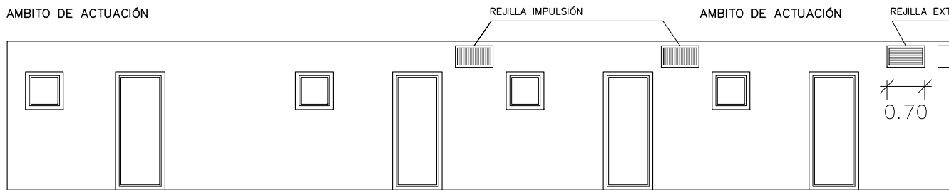
ALZADO (ESTADO FUTURO)
