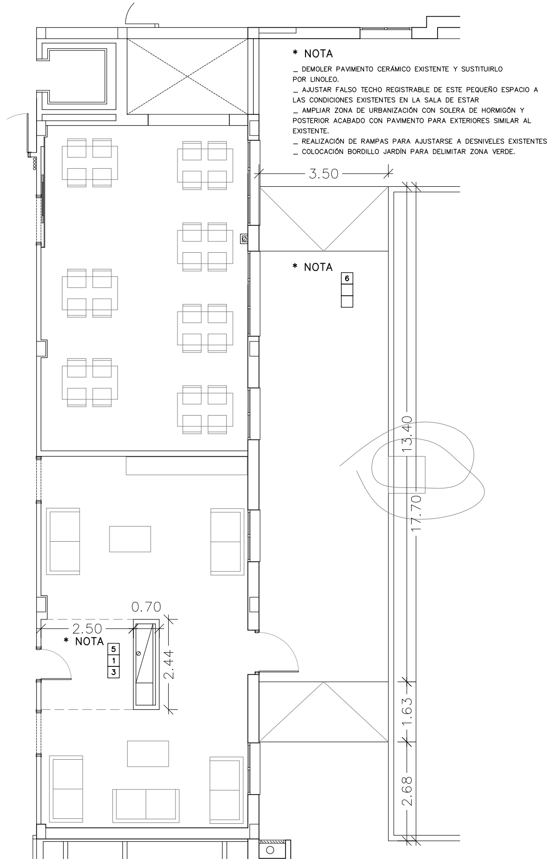
ACOTACIÓN FALSOS TECHOS ACABADOS Y ALTURAS
