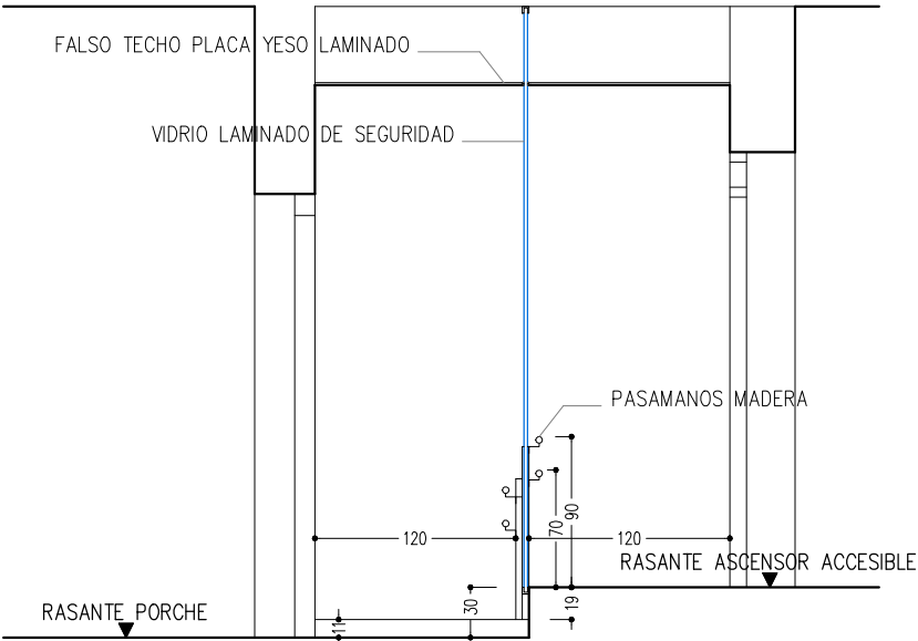
SECCIÓN TRANSVERSAL VESTÍBULO
