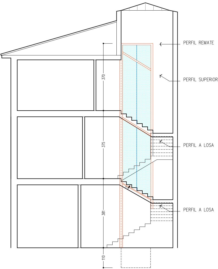
VISTA-SECCIÓN 2
