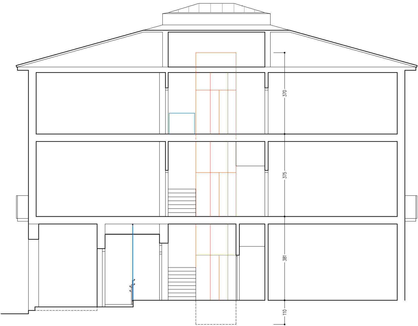
VISTA-SECCIÓN 1
