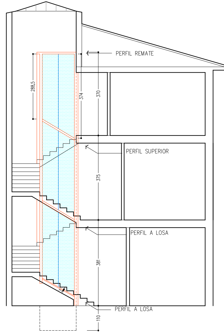
VISTA-SECCIÓN 4
