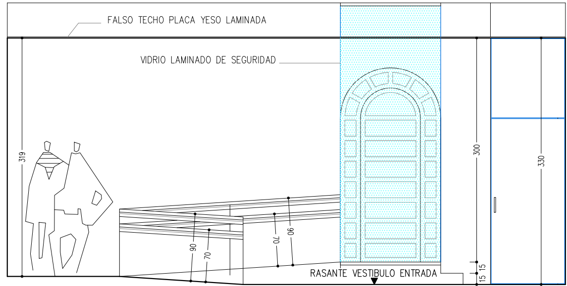
SECCIÓN LONGITUDINAL VESTÍBULO
