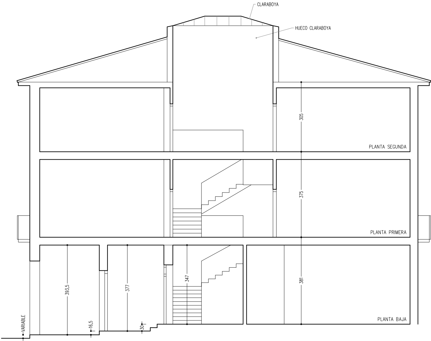
SECCIÓN GENERAL
