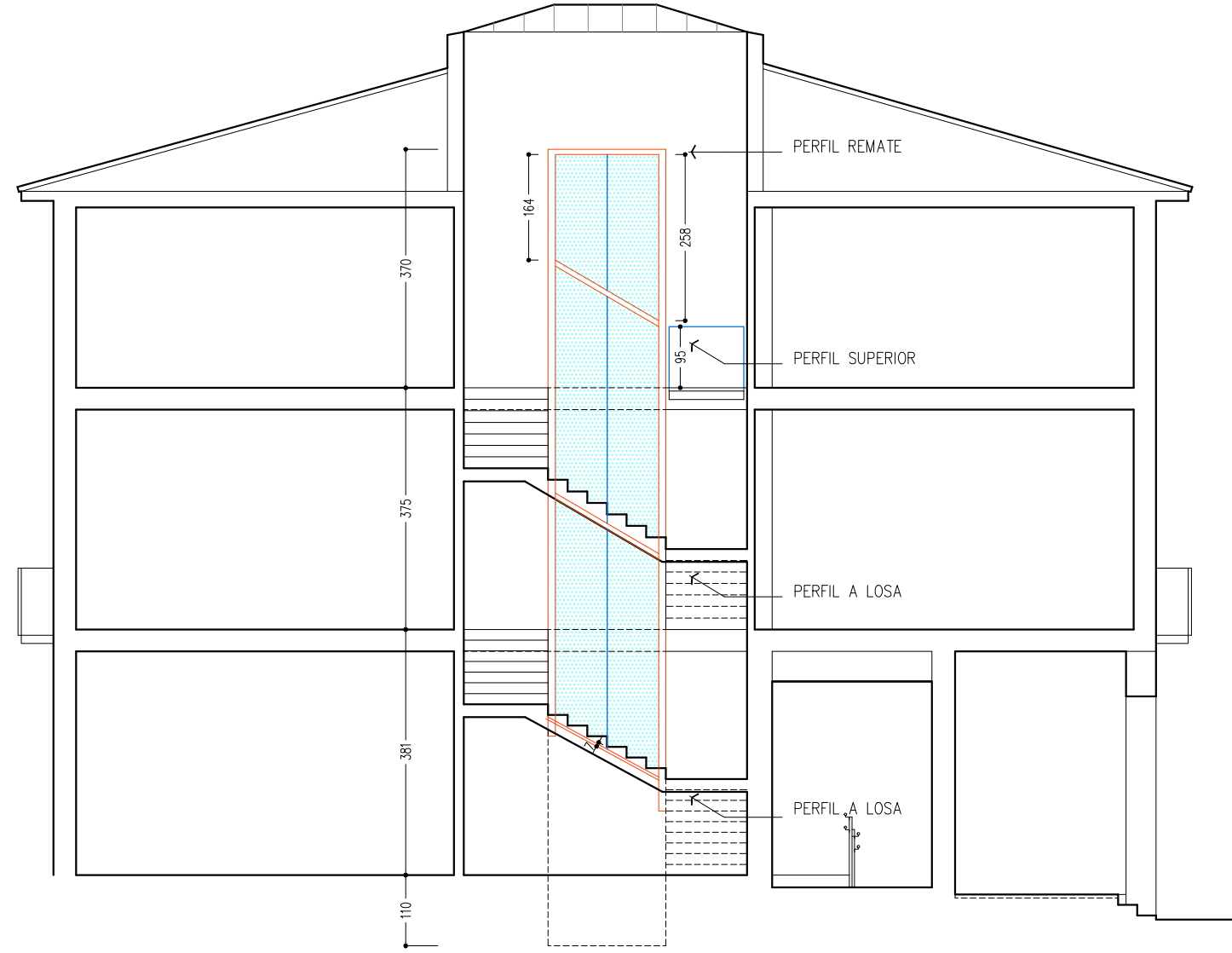
VISTA-SECCIÓN 3
